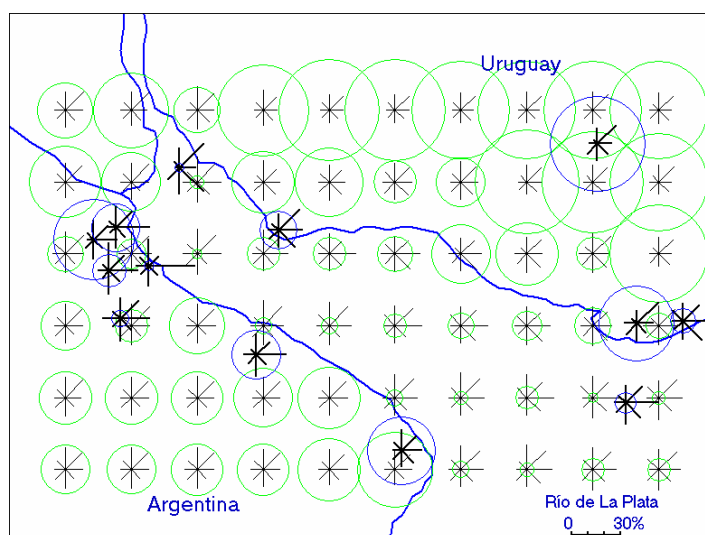
Figura 2 Frecuencia promedio de la dirección del viento obtenida con el modelo para el período 1994-2008
