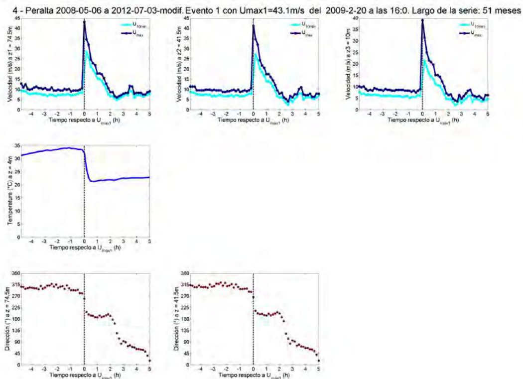
Figura 4: Evolución temporal de la velocidad, temperatura y dirección del viento durante dos tipos de eventos que producen las mayores ráfagas sobre Uruguay
