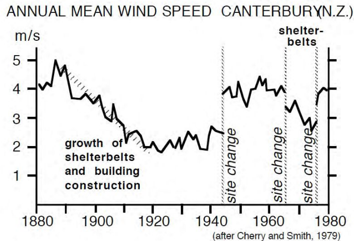
Figura 1: Variación de la velocidad media anual en una estación debido a cambios en su entorno y en su localización
