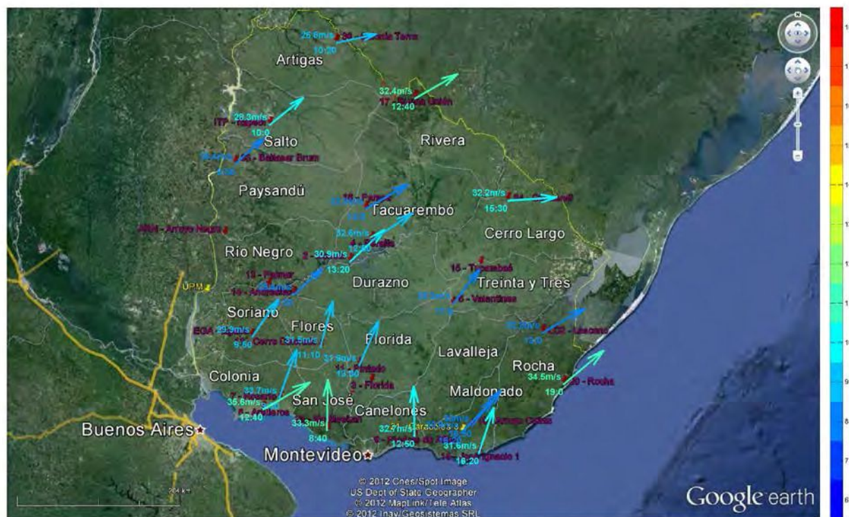
Figura 5: Algunos tipos de eventos que producen ráfagas intensas sobre Uruguay
