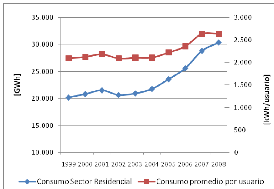
Figura 1. Evolución del consumo de electricidad del sector residencial. [Secretaría de Energía, 2009]
