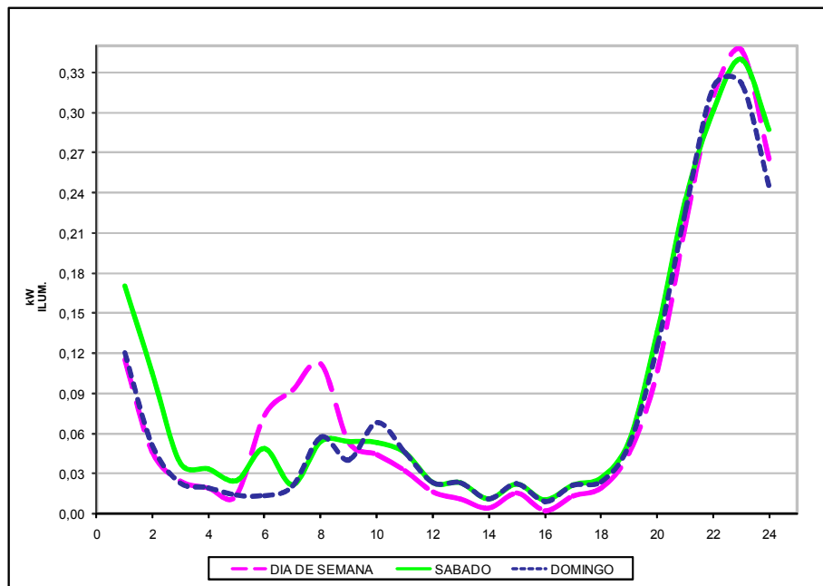
Figura 3. Curvas de carga del consumo eléctrico promedio en iluminación residencial obtenidas de la muestra de 17 casas del sector residencial de la región de C.A.B.A. y Gran Buenos Aires. Año 2008.
