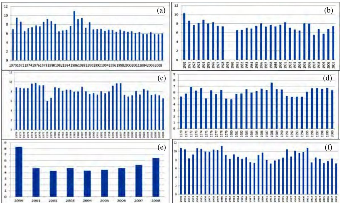
Figura 8- Velocidades medias anuales: (a) Río Gallegos, (b) Puerto Santa Cruz, (c) Puerto San Julián, (d) El Calafate (Aeropuerto Viejo), (e) El Calafate (Aeropuerto Nuevo), (f) Gobernador Gregores.
