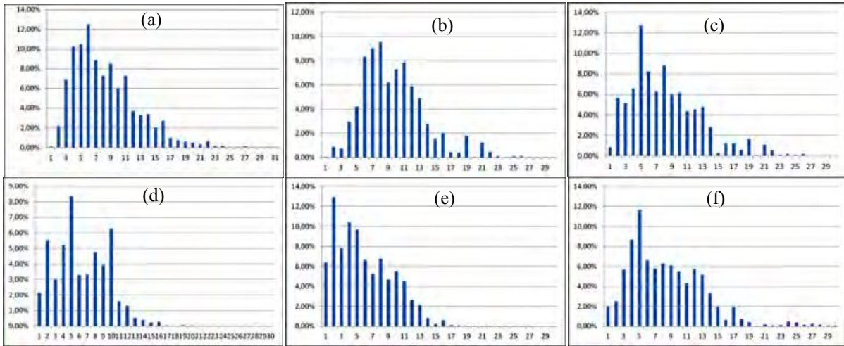
Figura 5- – Distribución de intensidades de vientos [m/s]: (a) Río Gallegos, (b) Puerto Santa Cruz, (c) Puerto San Julián, (d) El Calafate (Aeropuerto Viejo), (e) El Calafate (Aeropuerto Nuevo), (f) Gobernador Gregores.
