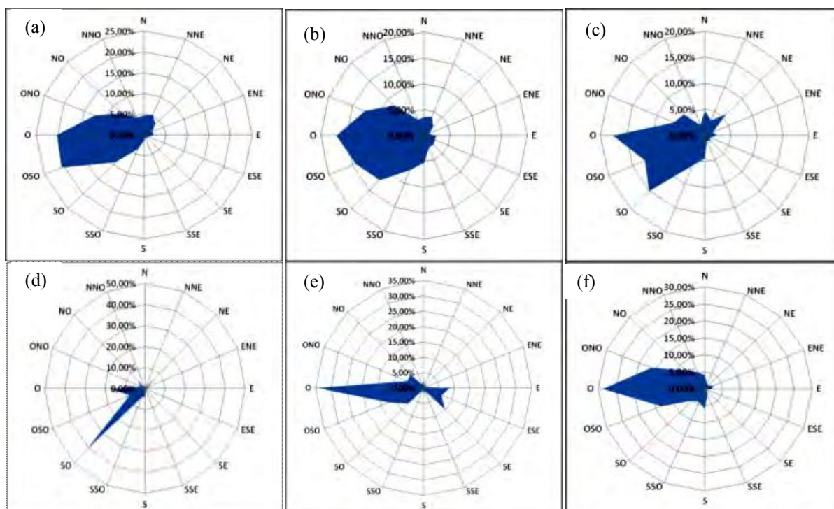
Figura 2- Rosas de Vientos anuales. (a) Río Gallegos, (b) Puerto Santa Cruz, (c) Puerto San Julián, (d) El Calafate (Aeropuerto Viejo), (e) El Calafate (Aeropuerto Nuevo), (f) Gobernador Gregores.
