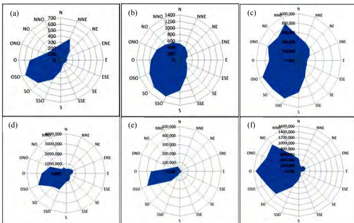
Figura 4- Rosas de Vientos anual de intensidades, con velocidades cúbicas [ m^3/s^3 ], para: (a) Río Gallegos, (b) Puerto Santa Cruz, (c) Puerto San Julián, (d) El Calafate (Aeropuerto Viejo), (e) El Calafate (Aeropuerto Nuevo), (f) Gobernador Gregores.
