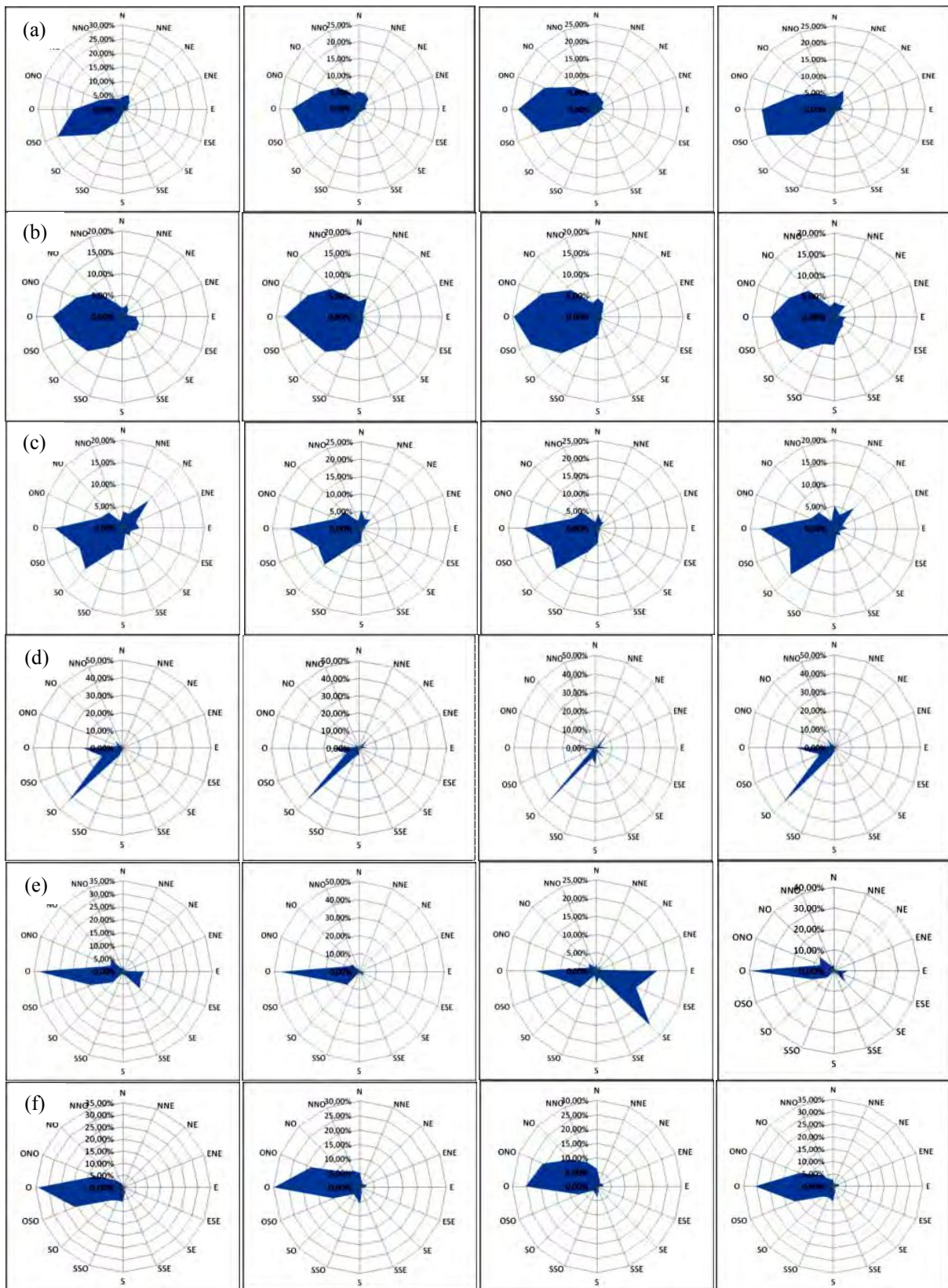
Figura 3- Rosas de Vientos estacionales, correspondientes a los meses de Enero, Abril, Julio y Octubre, para: (a) Río Gallegos, (b) Puerto Santa Cruz, (c) Puerto San Julián, (d) El Calafate (Aeropuerto Viejo), (e) El Calafate (Aeropuerto Nuevo), (f) Gobernador Gregores.
