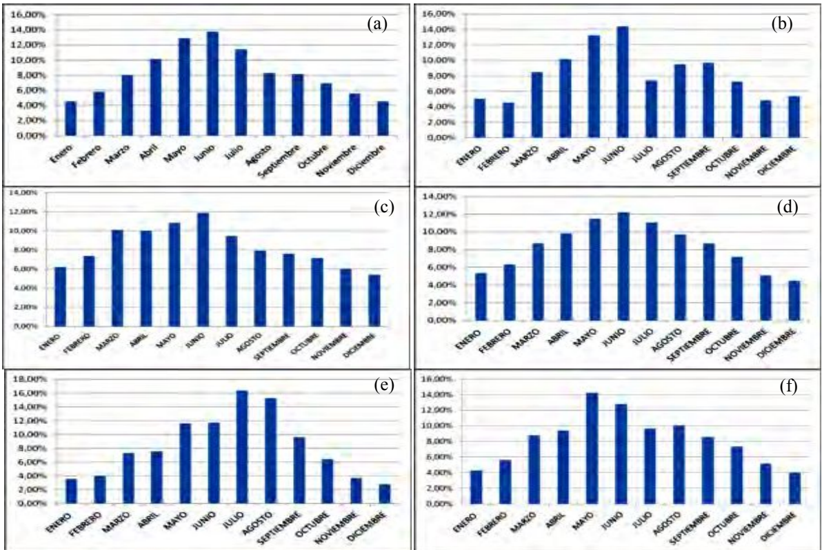
Figura 7- Porcentaje mensual de horas con calmas: (a) Río Gallegos, (b) Puerto Santa Cruz, (c) Puerto San Julián, (d) El Calafate (Aeropuerto Viejo), (e) El Calafate (Aeropuerto Nuevo), (f) Gobernador Gregores.
