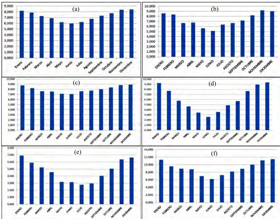
Figura 6- Distribuciones mensuales de intensidades de viento [m/s]: (a) Río Gallegos, (b) Puerto Santa Cruz, (c) Puerto San Julián, (d) El Calafate (Aeropuerto Viejo), (e) El Calafate (Aeropuerto Nuevo), (f) Gobernador Gregores.
