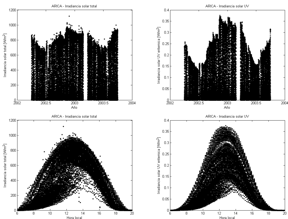
Figura 1. Mediciones de irradiancia solar total (izquierda) y UVE (derecha) en Arica durante los años 2002-2003 en función del día del año (superior) y de la hora local (inferior), en días cuyas tardes permanecieron mayormente despejadas.
