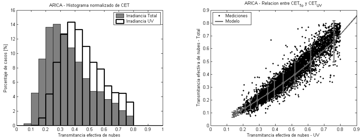
Figura 5. Izquierda: Histogramas de la transmitancia efectiva de nubes (CET) de la figura 4 en rango total (barras grises) y UVE (barras de contorno negro). Derecha: relación entre CET en rango total ( CET_{T0} ) y UVE ( CET_{UV} ) a partir de mediciones (puntos) y de cálculos con modelos (líneas), las barras de incerteza se deben al rango de SZA considerados.
