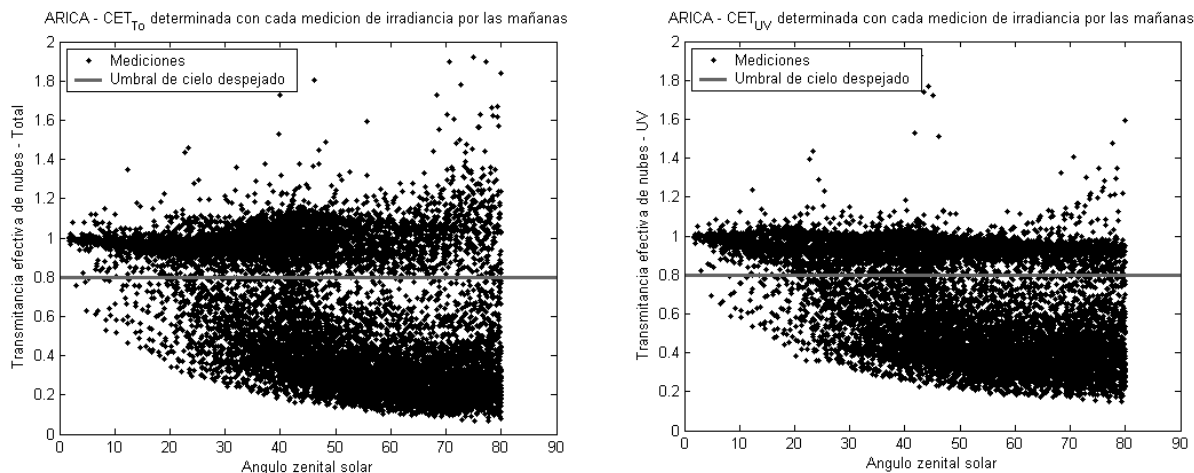
Figura 3. Transmitancia efectiva de nubes (CET) determinada a partir de cada medición de irradiancia solar en rango total (izquierda) y UVE (derecha) en función del ángulo zenital solar.
