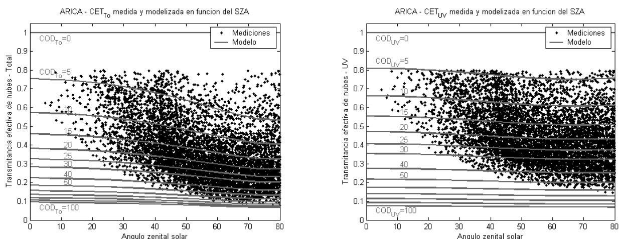
Figura 4. Transmitancia efectiva de nubes (CET) para condiciones de nubosidad ( \text{CET} < 0.80 ) extraídas de la figura 3 en rango total (izquierda) y UVE (derecha) en función del ángulo zenital solar. Las líneas grises representan la CET modelizada en función del ángulo zenital solar para espesores ópticos de nubes (COD) desde 0 a 100 en ambos rangos. Se seleccionaron datos correspondientes a \text{SZA} < 80^\circ .
