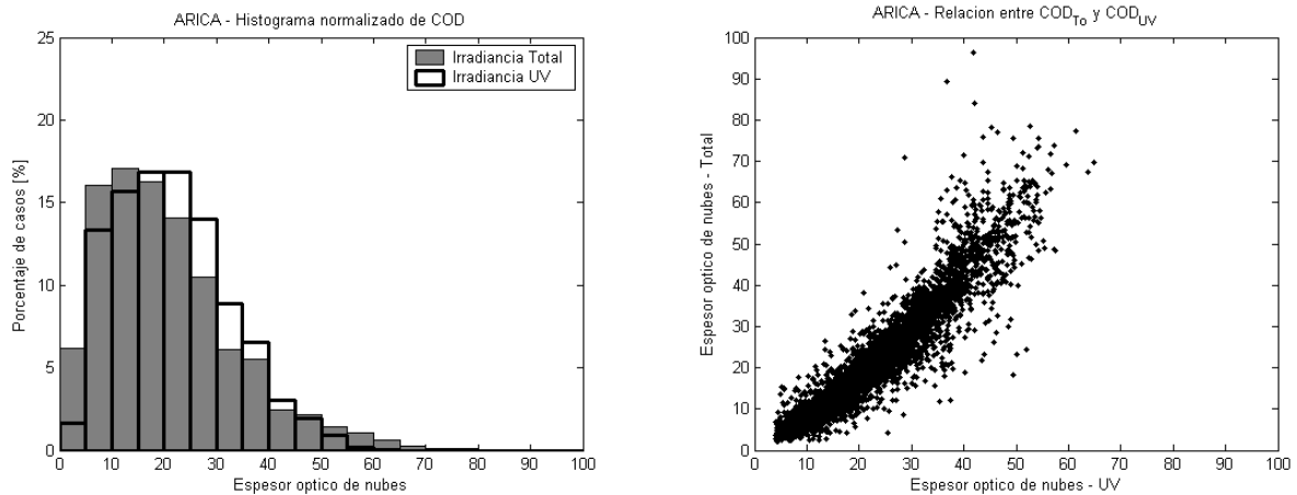
Figura 6. Izquierda: Histogramas del espesor óptico de nubes (COD) determinados a partir de la figura 4 en rango total (barras grises) y UVE (barras de contorno negro). Derecha: relación entre COD en rango total ( COD_{T0} ) y UVE ( COD_{UV} ) a partir de las mediciones.
