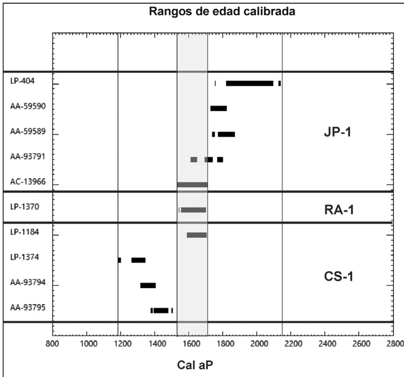
Figura 2. Fechados radiocarbónicos calibrados con CALIB 7.1 (Stuiver et al. 2017) sobre restos humanos de los sitios JP-1, RA-1 y CS-1. El sector en gris indica el superlapiamiento temporal máximo de los tres sitios.
