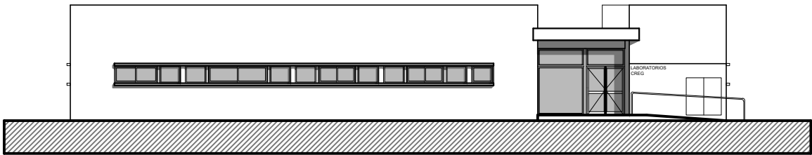
VISTA SUR
