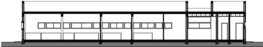
CORTE LONGITUDINAL
