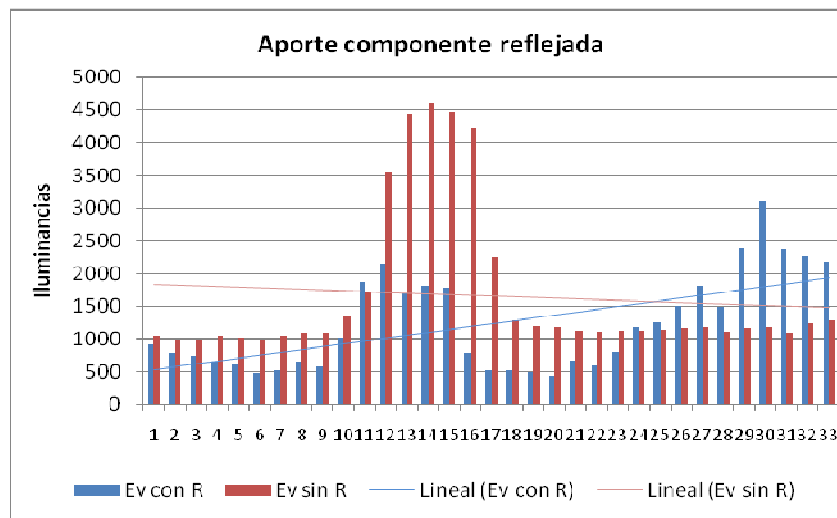
Figura 11: Barras comparativas de Iluminancias con y sin presencia de fachada captora para 16m.
