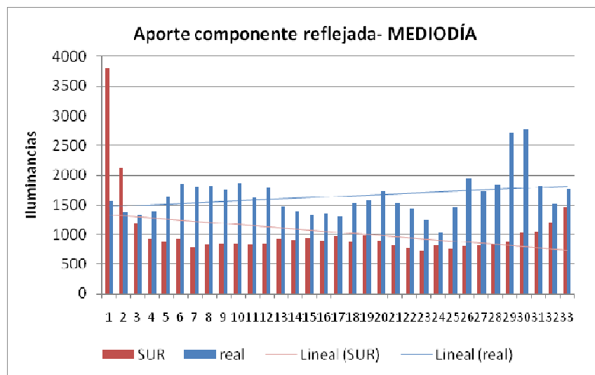
Figura 9: Barras comparativas de Iluminancias con y sin presencia de fachada captora para 20m.
