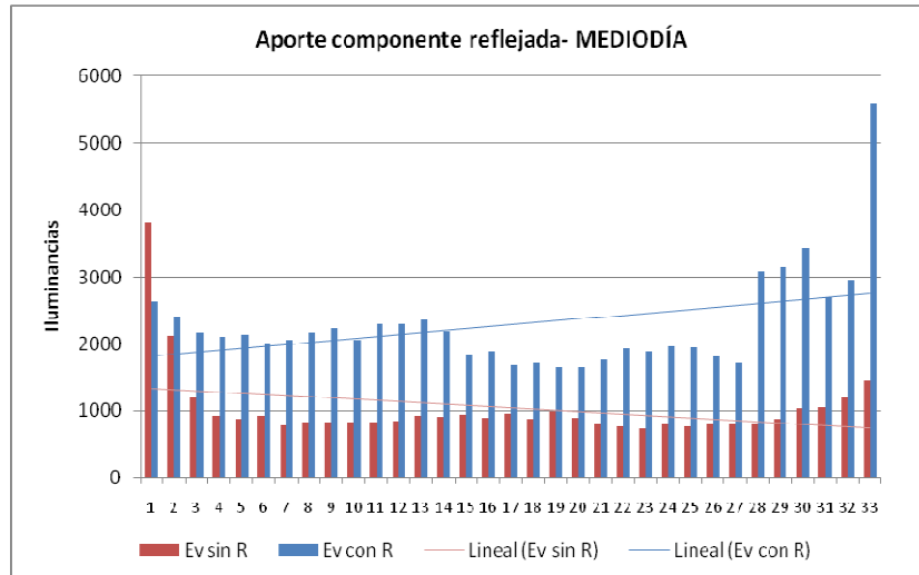
Figura 7: Barras comparativas de Iluminancias con y sin presencia de fachada captora para 30m.
