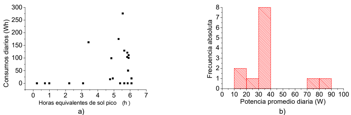
Figura 1: Datos registrados durante el primer periodo en la zona escuela. a) Consumos diarios registrados únicamente de lunes a viernes, en función de las horas equivalentes de sol pico correspondientes. b) Distribución de las 13 potencias diarias no-nulas registradas.
