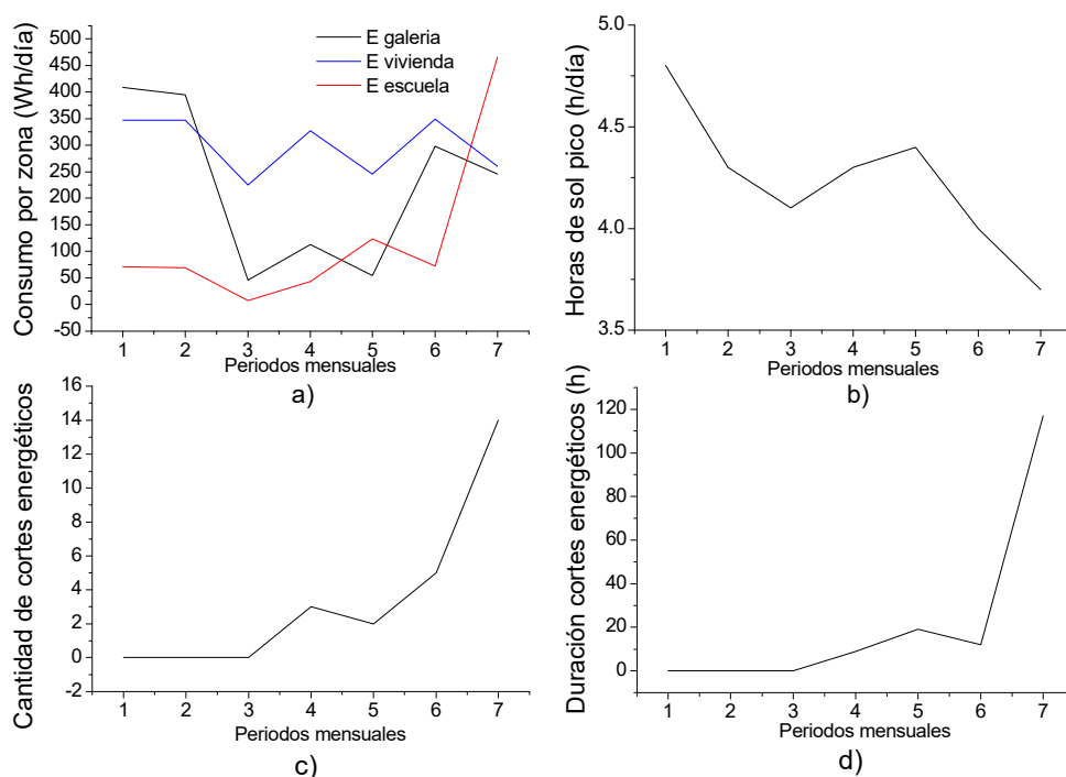
Figura 4: Promedios mensuales de datos registrados durante un total de 7 periodos.
