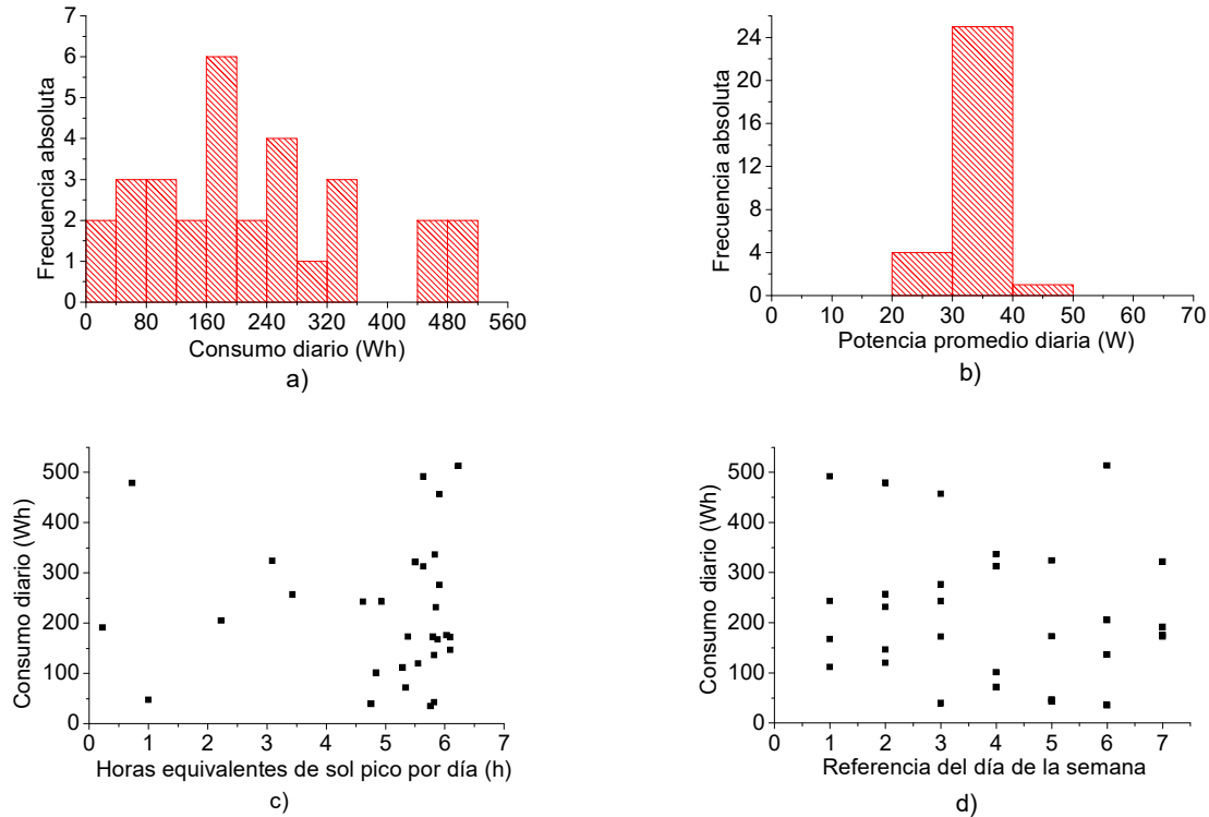
Figura 2: Distribución de a) consumos, b) potencias diarios registrados durante el primer periodo en la zona vivienda. Consumos diarios en función de c) las horas equivalentes de sol pico correspondientes y d) del día de la semana (el día lunes está referenciado por ser el día 1, el domingo el día 7).
