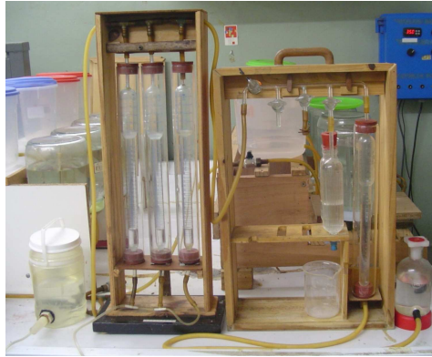
Figura 2: Imagen del conjunto de cuantificación de biogás y CO 2 , respectivamente las tres buretas y el aparato ORSAT. Atrás y a la izquierda la unidad de generación, al fondo a la derecha: el tablero de control.
