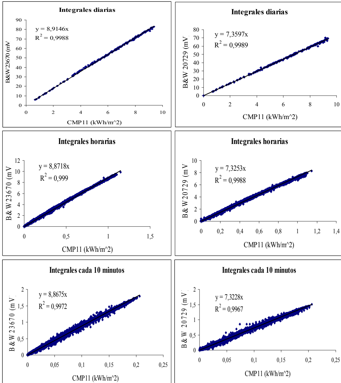
Figura 7: Calibración mediante la comparación de las integrales diarias, horarias y cada 10 minutos con un patrón secundario Kipp&Zonnen CMP11
