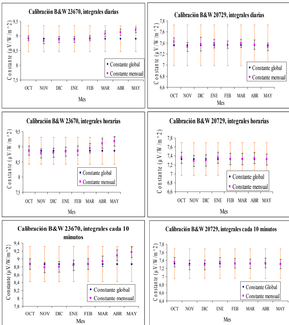
Figura 8: Constantes de calibración por mes con el error asociado (barras color negro), constante de calibración global, error arbitrario de 5 % asociado a la constante global (barras color naranja)
