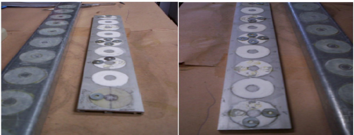
Figura 6: Probetas para el ensayo de adherencia
