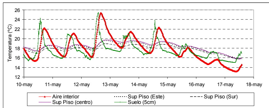
Figura 4. Temperatura del aire interior del prototipo, temperatura del suelo a 5cm de profundidad y temperatura superficial del piso en el centro y laterales Este y Sur del prototipo.
