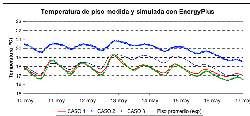
Figura 8. Temperatura de la superficie del piso simulada con EnergyPlus y medida experimentalmente, para tres posibilidades de simulación del piso.
