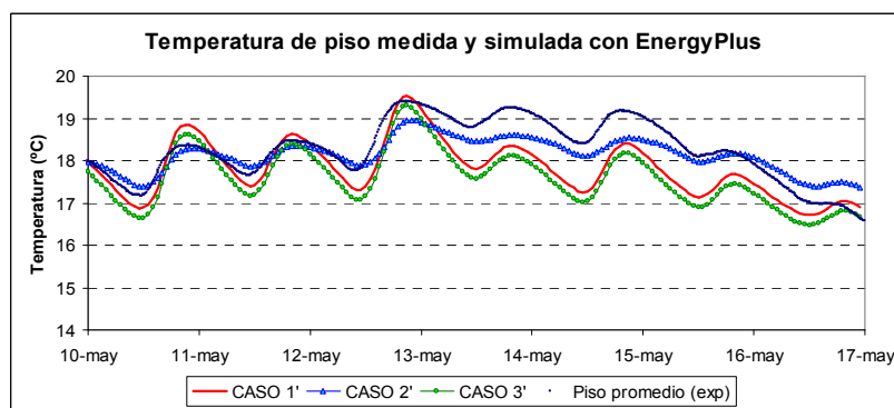
Figura 9. Temperatura de la superficie del piso simulada con EnergyPlus y medida experimentalmente, para las tres posibilidades de simulación del piso, con un mes previo de simulación.
