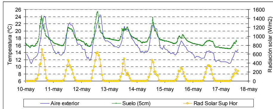
Figura 3. Temperatura del aire exterior, temperatura del suelo a 5cm de profundidad y radiación solar sobre superficie horizontal, para el periodo comprendido entre el 10 y el 17 de mayo de 2011.
