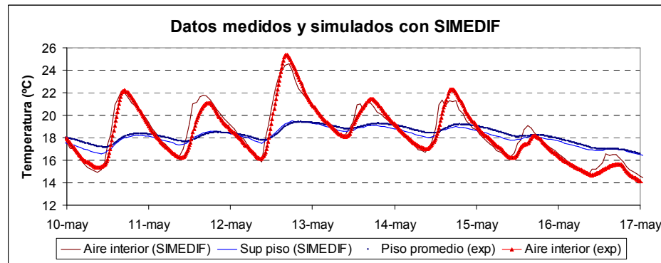
Figura 5. Temperatura del aire interior y temperatura superficial del piso del prototipo, medida y simulada con SIMEDIF para el periodo comprendido entre el 10 y el 17 de mayo de 2011.
