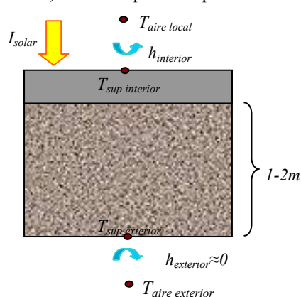
Figura 1. Modelización del piso en SIMEDIF
