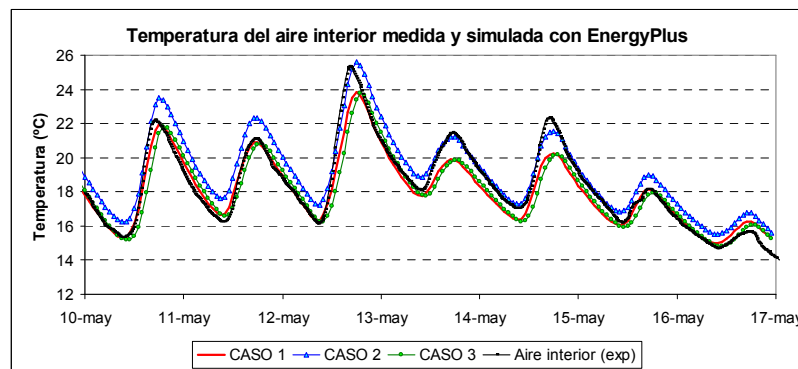
Figura 7. Temperatura del aire interior del prototipo simulada con EnergyPlus y medida experimentalmente, para tres posibilidades de simulación del piso.
