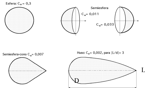
Fig. 3.5.- Coeficiente k para algunos perfiles semiesféricos
