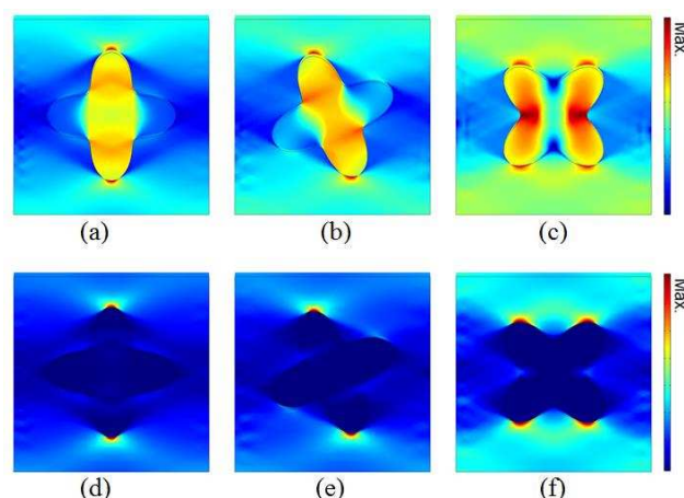
Figura 12: Campos de tensión y deformación equivalentes cuando la celda alcanza una deformación \varepsilon_y = 0.02 con condición de contorno del caso C: Tensión de Von Mises para (a) \theta_0 = 0^\circ , (b) \theta_0 = 22.5^\circ y (c) \theta_0 = 45^\circ ; Deformación plástica equivalente para (d) \theta_0 = 0^\circ , (e) \theta_0 = 22.5^\circ y (f) \theta_0 = 45^\circ .
