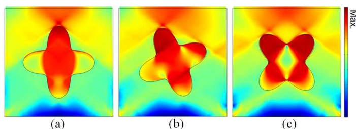
Figura 11: Tensión equivalente de Von Mises cuando la celda alcanza una deformación \varepsilon_y = 0.02 con condición de contorno del caso A: (a) \theta_0 = 0^\circ , (b) \theta_0 = 22.5^\circ y (c) \theta_0 = 45^\circ .
