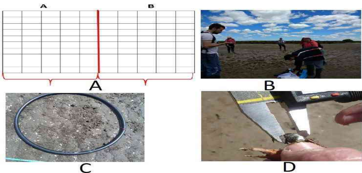
Figura 4: Muestreo de Uca uruguayensis . A y B: Esquema y colocación de cuadrículas utilizadas para el muestreo. C: unidad muestral del muestreo sistemático. D: medición de la longitud del cefalotórax de Ucauruguayensis con calibre Vernier.
