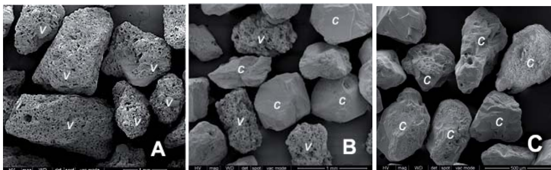
Figura 6. Fotomicrografía SEM correspondiente a: A) P_3 : Fracción >1 mm, donde se observan vitroclastos (v), B) P_4 : fracción de 0,5-1 mm, donde se observan vitroclastos (v) y cristaloclastos © y C) P_5 : fracción de 0,25-0,5 mm, con presencia de cristaloclastos.
