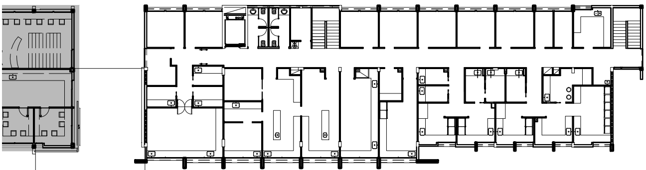
PLANTA SEGUNDA
