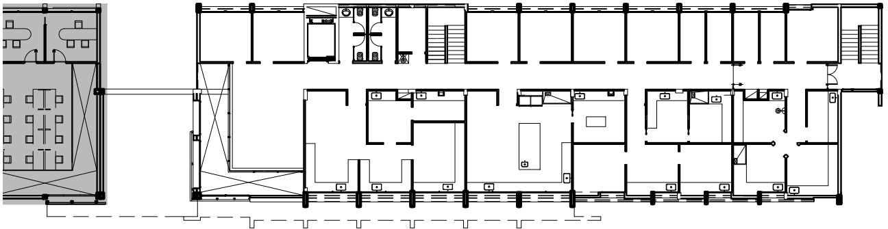
PLANTA PRIMERA
