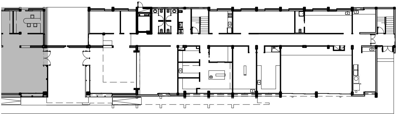
PLANTA BAJA
