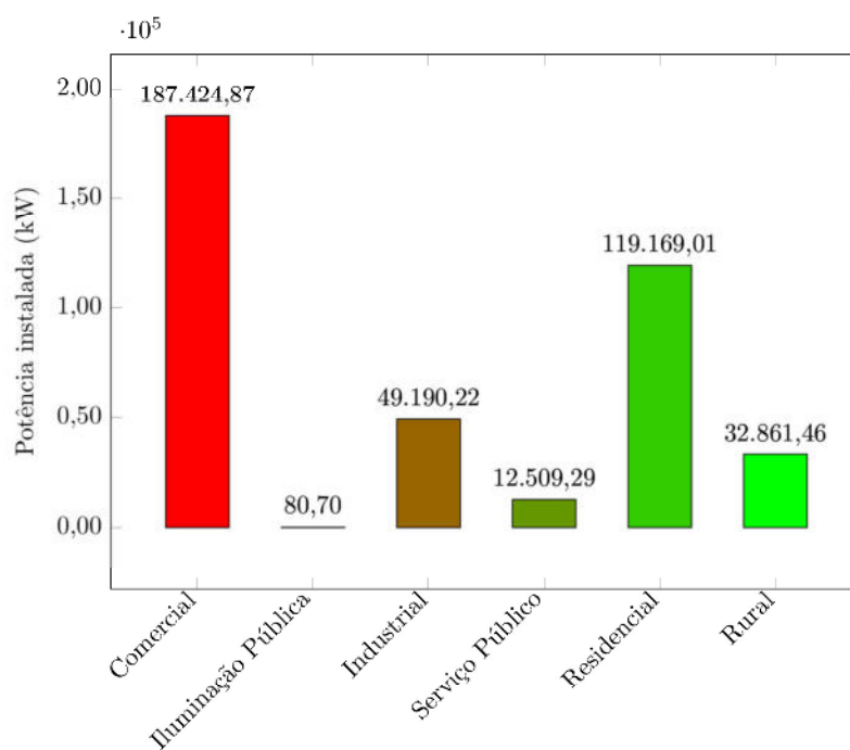
Figura 11 - Potências dos sistemas em GD instalados até julho de 2018 no Brasil por classe de consumo.
