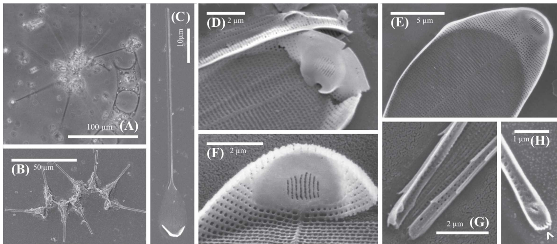
Fig. 2: Asterionellopsis glacialis . (A): MO. (B-H): MEB. (A) y (B): aspecto general de las colonias. (C) Valva heteropolar, espátuliforme. (D) Polo basal de la valva en vista externa con parte de una banda. (E) Polo basal de la valva en vista interna. (F) Vista interna del campo apical de poros atravesado por costillas. (G) A la derecha polo apical de la valva en vista externa mostrando la abertura del proceso labiado y las espinas ubicadas en la unión superficie valvar y manto. A la izquierda polo apical en vista interna inclinada. (H) Polo apical de la valva en vista interna mostrando el proceso labiado cercano al campo apical de poros (flecha).
