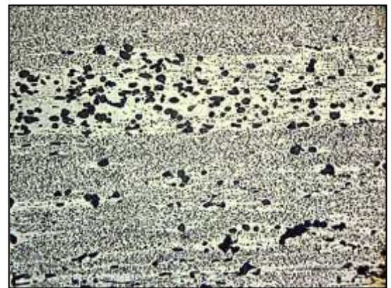
Figura 14 – Micrografía de la muestra con recocido de ablandamiento hasta 290 °C y temple, con un 85,7 % de deformación acumulada, 200x.
