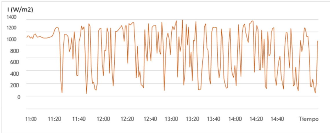
Figura 8: Irradiancia minutil ( W/m^2 ) entre las 11 y las 15 hs del día 4/12/2017 en la estación Balcarge
