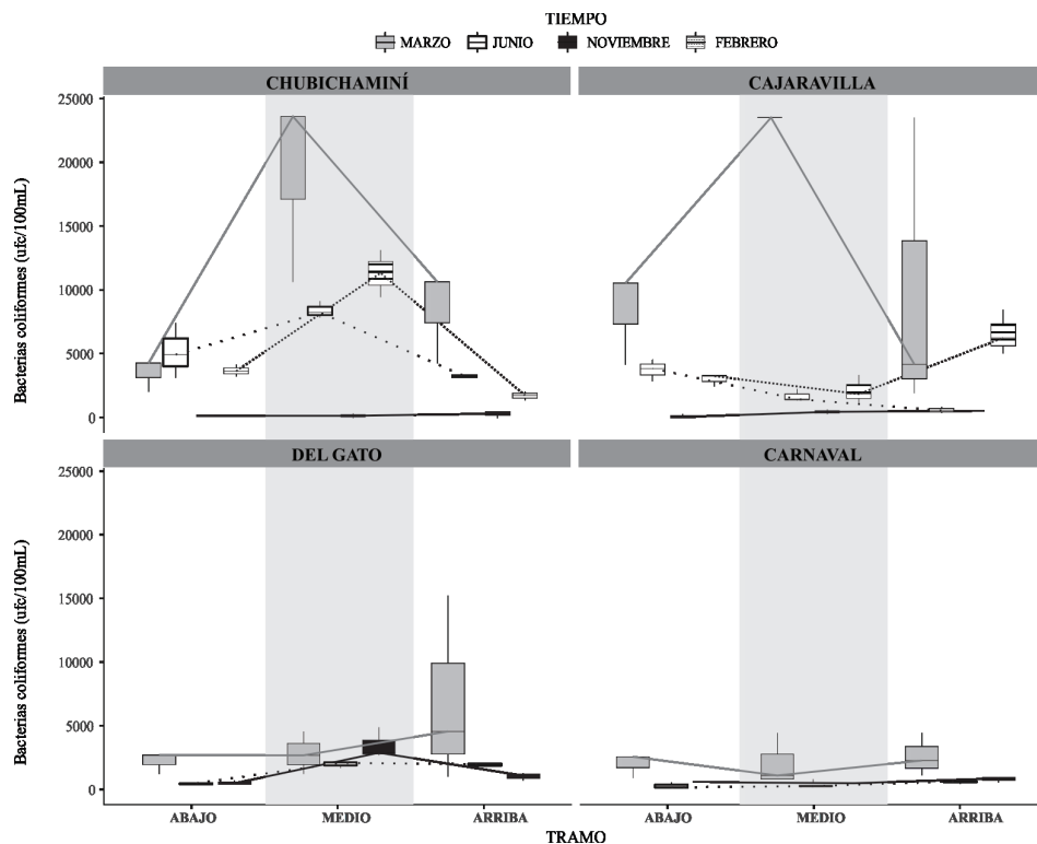
Figura 5. Variación en la densidad de bacterias coliformes fecales ( E. coli ) en los tres tramos de cada uno de los cuatro cauces en los períodos muestreados.
