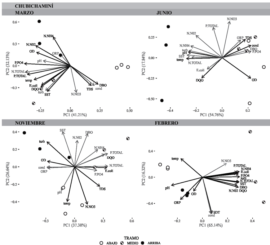
Figura 1. Resultados de los ACP para el cauce Chubichaminí, por cada período muestreado. Los vectores en negro representan aquellas variables significativas (MANOVA p < 0.05 ) para diferenciar los tres tramos (Abajo, Medio, Arriba) en cada momento del año.
