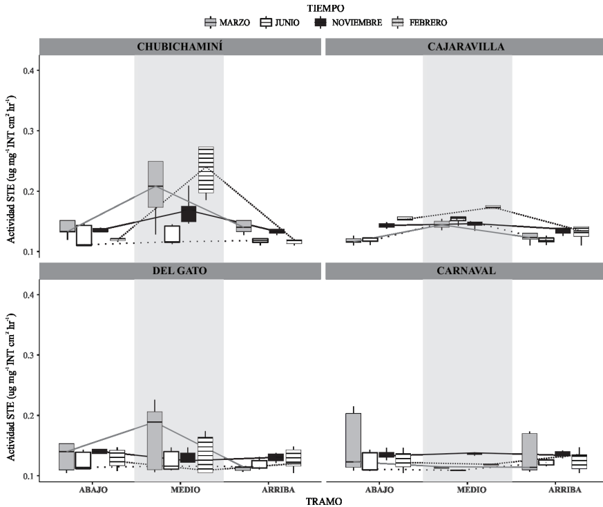
Figura 6. Variación de la actividad del sistema transportador de electrones (STE) en el sedimento de los tres tramos de los cuatro cauces en los períodos muestreados.
