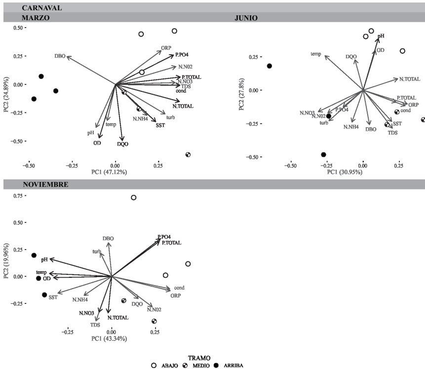
Figura 4. Resultados de los ACP para el cauce Carnaval, por cada período muestreado. Los vectores en negro representan aquellas variables significativas (MANOVA p < 0.05 ) para diferenciar los tres tramos (Abajo, Medio, Arriba) en cada momento del año.
