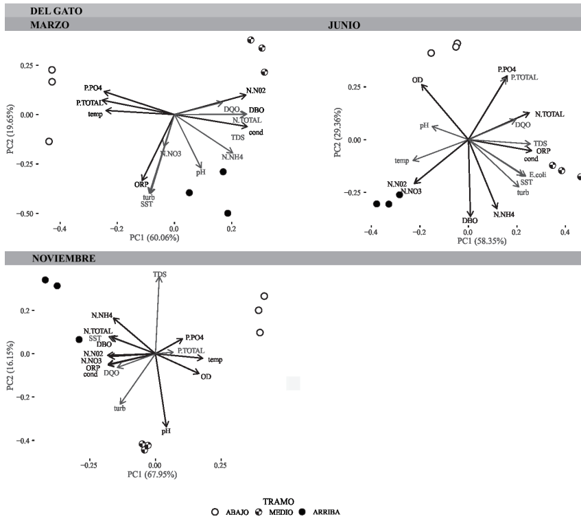
Figura 3. Resultados de los ACP para el cauce Gato, por cada período muestreado. Los vectores en negro representan aquellas variables significativas (MANOVA p < 0.05 ) para diferenciar los tres tramos (Abajo, Medio, Arriba) en cada momento del año.
