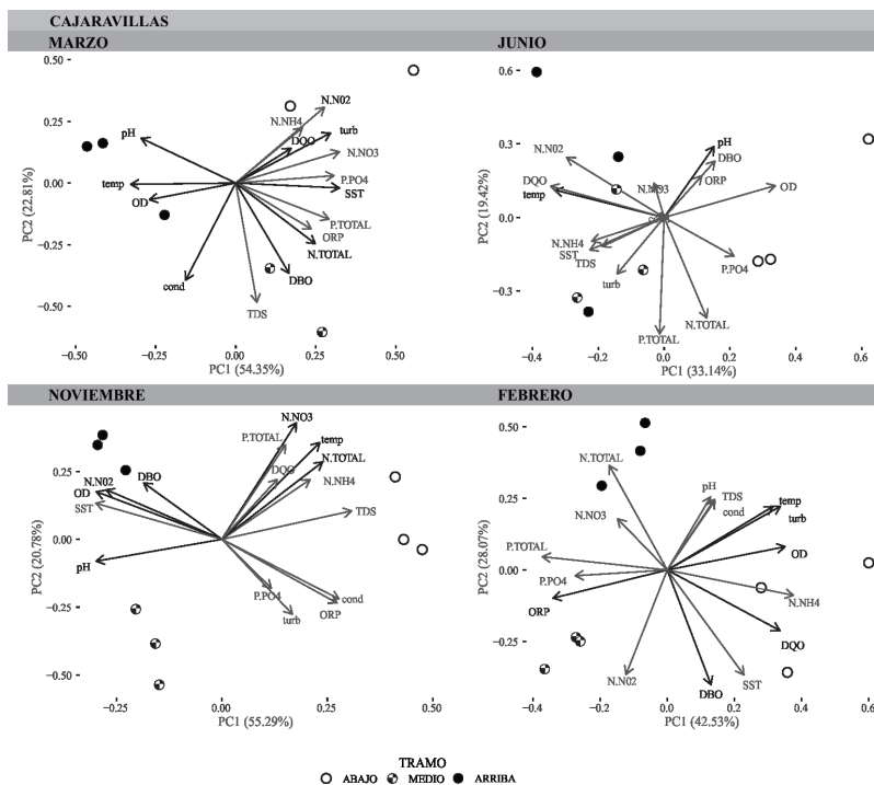
Figura 2. Resultados de los ACP para el cauce Cajaravillas, por cada período muestreado. Los vectores en negro representan aquellas variables significativas (MANOVA p < 0.05 ) para diferenciar los tres tramos (Abajo, Medio, Arriba) en cada momento del año.
