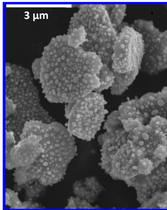
Nanopartículas de \text{Ni}^0 sobre la matriz oxídica
