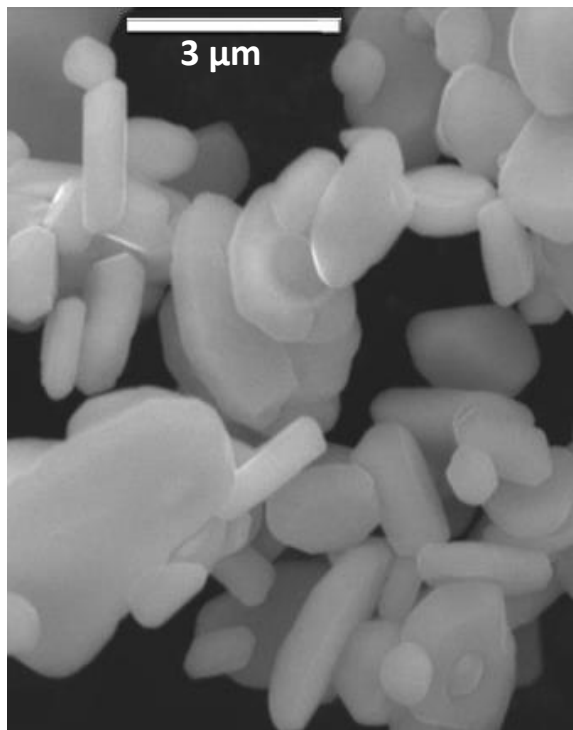
\text{NiTiO}_3 calcinado a 850^\circ\text{C}
