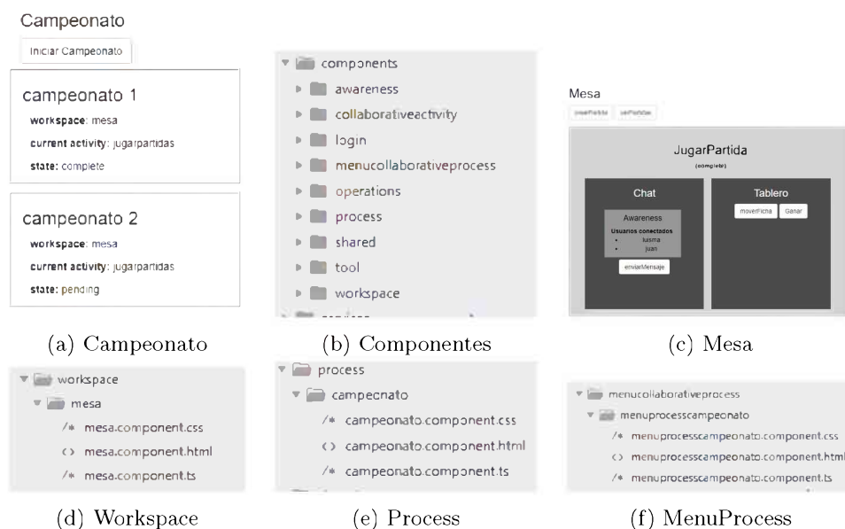
Figura 11: Estructura de la plataforma de implementación
