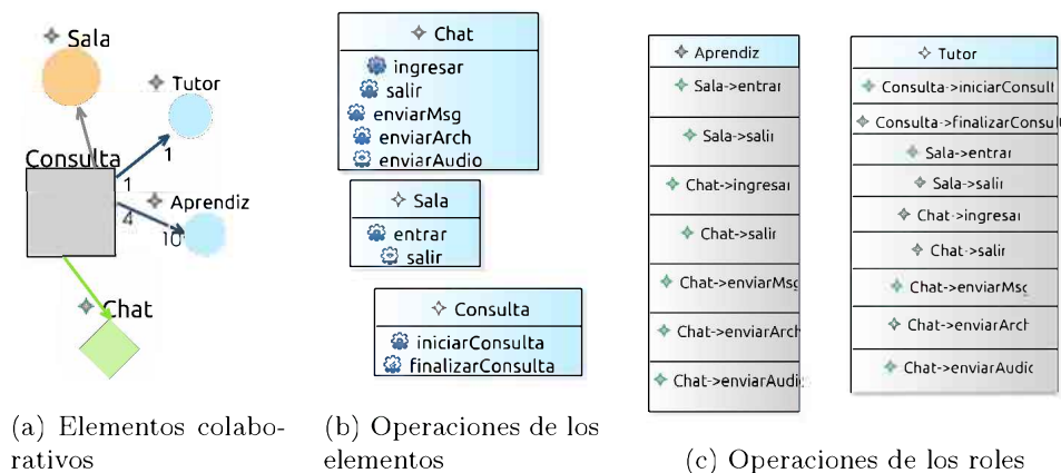
Figura 5: Modelo de un chat simple
