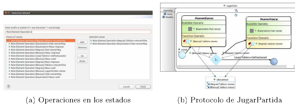
Figura 9: Protocolos de actividades colaborativas
