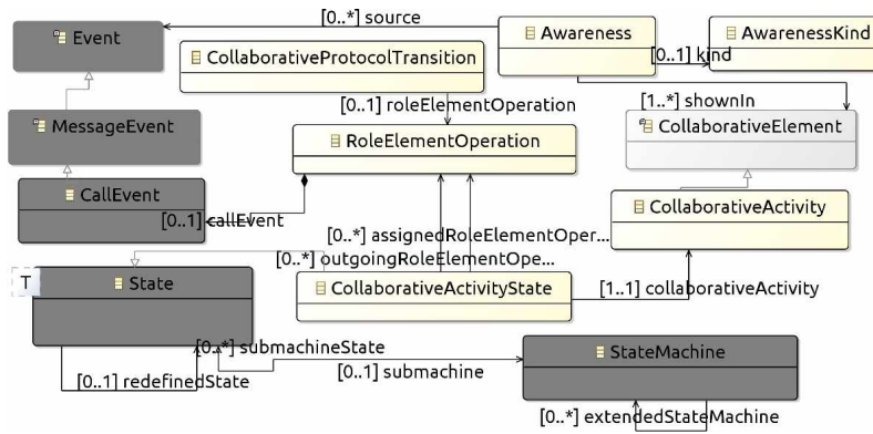
Figura 3: Modelo de Protocolos con Awareness
