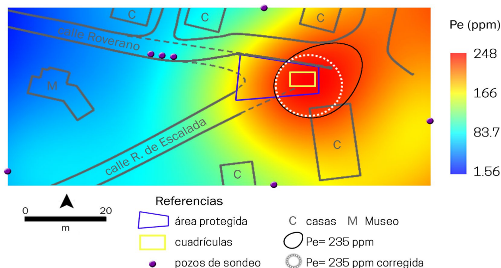
Figura 3. Modelo de distribución espacial de los valores de fósforo extraíble (Pe) en partes por millón (ppm), con indicación del perímetro calculado como límite del área de enterramiento sobre la base de 235 ppm de Pe y 235 ppm corrected .
