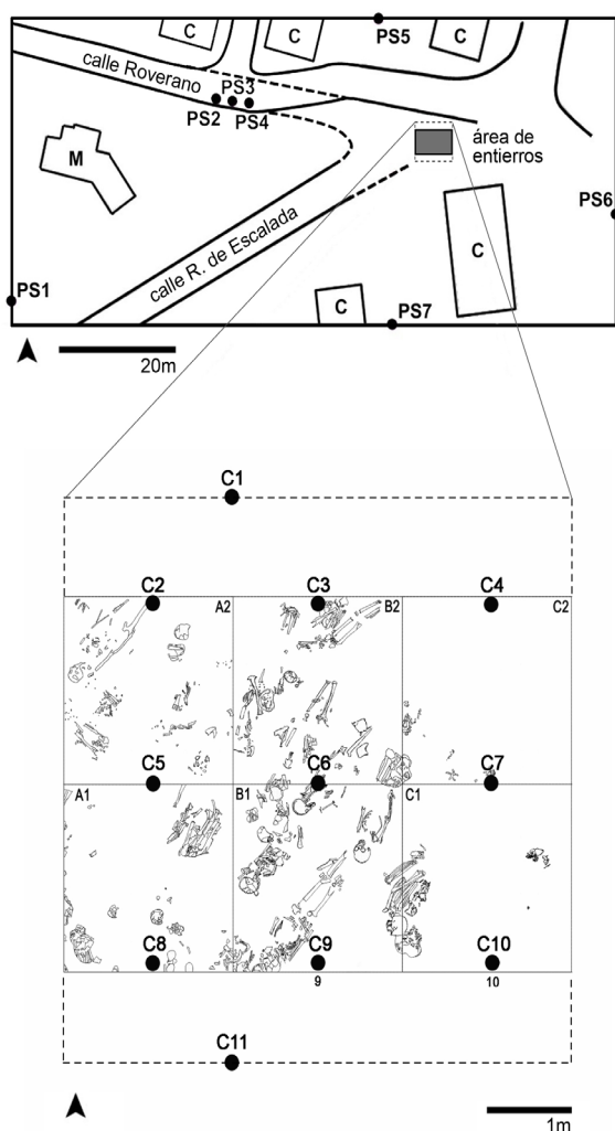
Figura 2. Localización del área de entierro del sitio RSCII y de las unidades de muestreo consideradas para el análisis químico del suelo (C1...C11= cuadrículas; PS1...PS7= pozos de sondeo).
