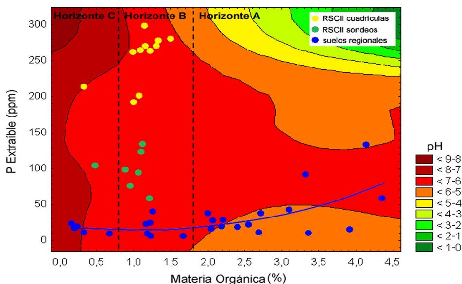
Figura 4. Diagrama de dispersión de los valores de Pe (ppm) en relación con los porcentajes de materia orgánica (%MO) y pH para muestras de suelo del sector de cuadrículas, de los pozos de sondeo y de los suelos regionales.
