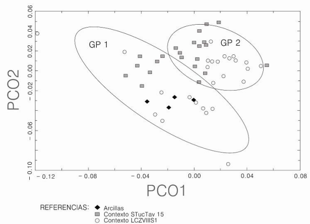
Figura 4. Agrupamiento de arcillas y fragmentos en el espacio factorial definido por los factores 1 y 2. n=54. Tomado de Páez y Plá (2015).
