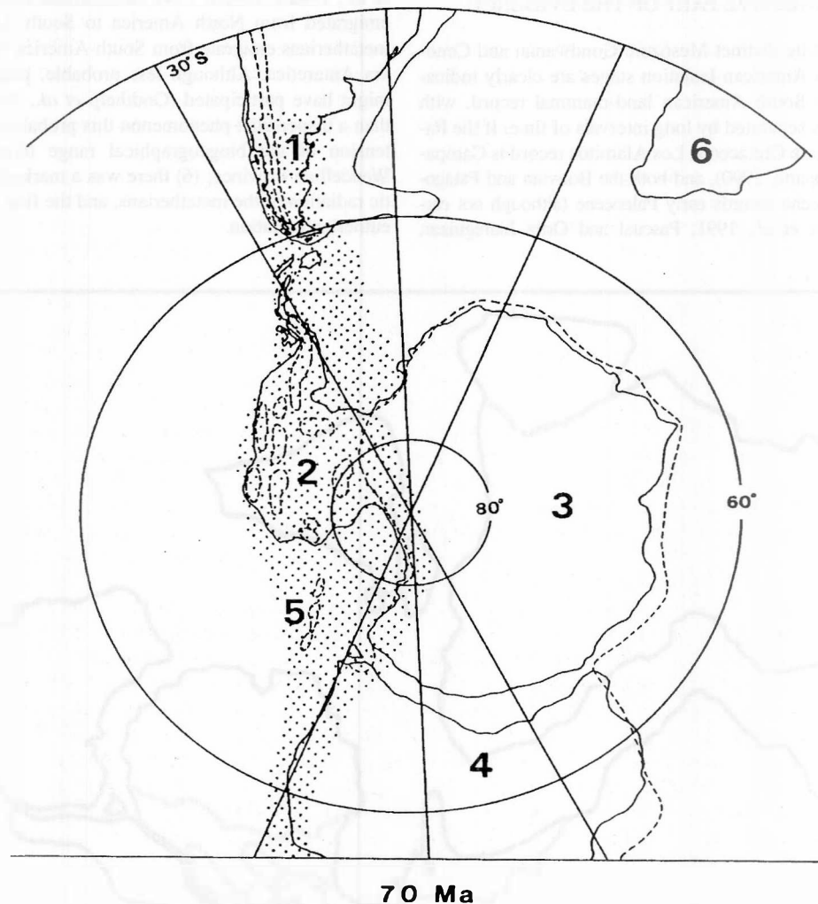
Figure 3. The paleobiogeographical Weddellian Province approximately between 70 and 61 Ma. (Modified from Zinsmeister, 1982, and Case, 1988). 1. Southern South America; 2. Western Antarctica; 3. Antarctic craton; 4. Australia; 5. New Zealand; 6. Southern Africa. The present South American Atlantic configuration was created later than the African, approximately by the late Paleogene. / La Provincia Weddelliana (biogeográfica) aproximadamente entre 70 y 61 Ma (Modificado de Zinsmeister, 1982 y de Case, 1988). 1. Sur de Sudamérica; 2. Antártida Occidental. 3. Cratón Antártico. 4. Australia. 5. Nueva Zelanda. 6. África del Sur. La configuración atlántica de Sudamérica fue creada más tarde que la de África, aproximadamente por el Paleógeno tardío.
