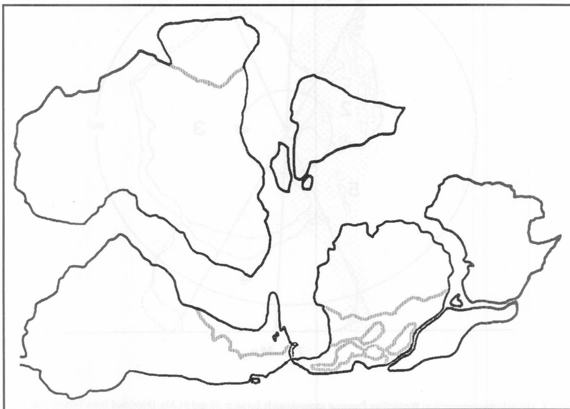
Figure 2. Gondwanaland reconstruction for 100 Ma. The present African Atlantic configuration had already been created. Gray line: present coast line; black line: past coast line (modified from Storey, 1995). / Reconstrucción del supercontinente de Gondwana a los 100 Ma. La actual configuración atlántica de África habíase creado ya. Línea gris: línea de costas actuales. Línea negra: línea de costas a los 100 Ma (modificado de Storey, 1995).
