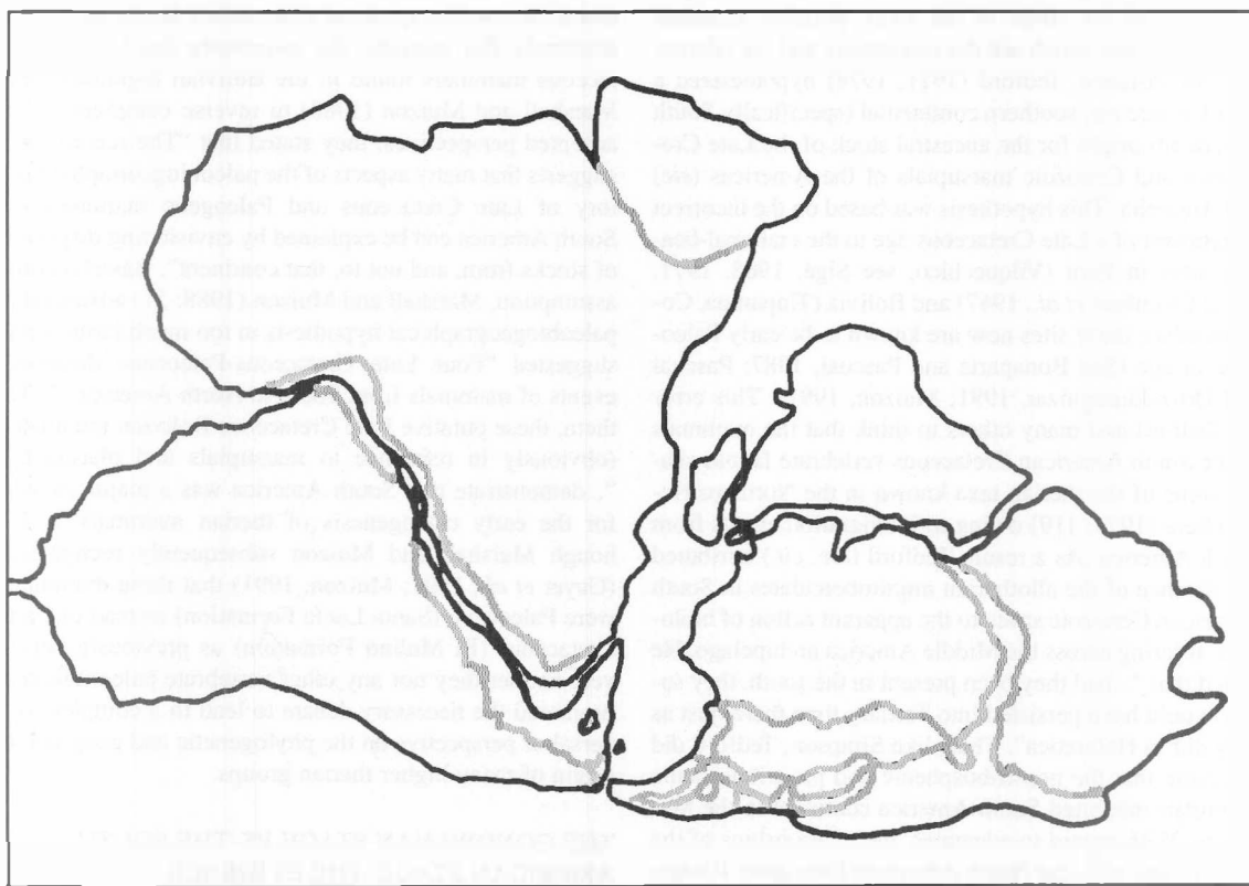
Figure 1. Gondwanaland reconstruction for 130 Ma. The South Atlantic opened earlier than the Equatorial Atlantic. Gray line: present coast line; black line: past coast line (modified from Storey, 1995.) / Reconstrucción del supercontinente de Gondwana a los 130 Ma. El Atlántico sur se abrió antes que el Atlántico ecuatorial. Línea gris: línea de las costas actuales. Línea negra: línea de costas a los 130 Ma (modificado de Storey, 1995).
