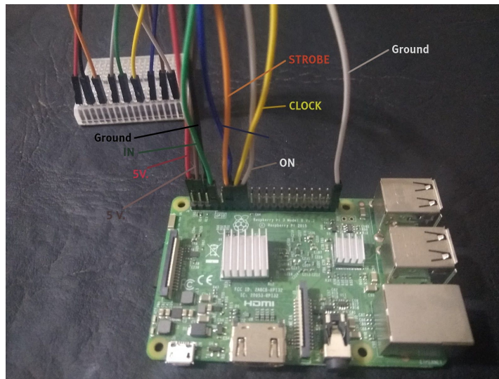
Fig. 6. Ejemplo de cómo debe quedar la instalación en nuestra Raspberry PI
