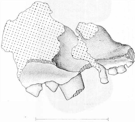
Figura 3. Hondonadia feruglioi n. gen. et sp. MPEF-PV 1004 (holotipo), porción rostral con parte del premaxilar y el maxilar, incluyendo cuatro incisivos, el canino y los dos primeros premolares; vista lingual. Escala: 1 mm. / MPEF-PV 1004 (holotype), facial part of a skull including parts of the premaxilla and maxilla, four incisors, the canine, and the first two premolars, lingual view. Scale: 1 mm.
