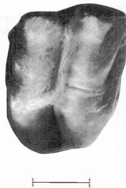
Figura 4. Hondonadia feruglioi n. gen. et sp. MPEF-PV 1004 (holotipo), M?1 izquierdo, aislado; vista oclusal. Escala: 1 mm. / MPEF-PV 1004 (holotype), isolated left M?1, occlusal view. Scale: 1 mm.
