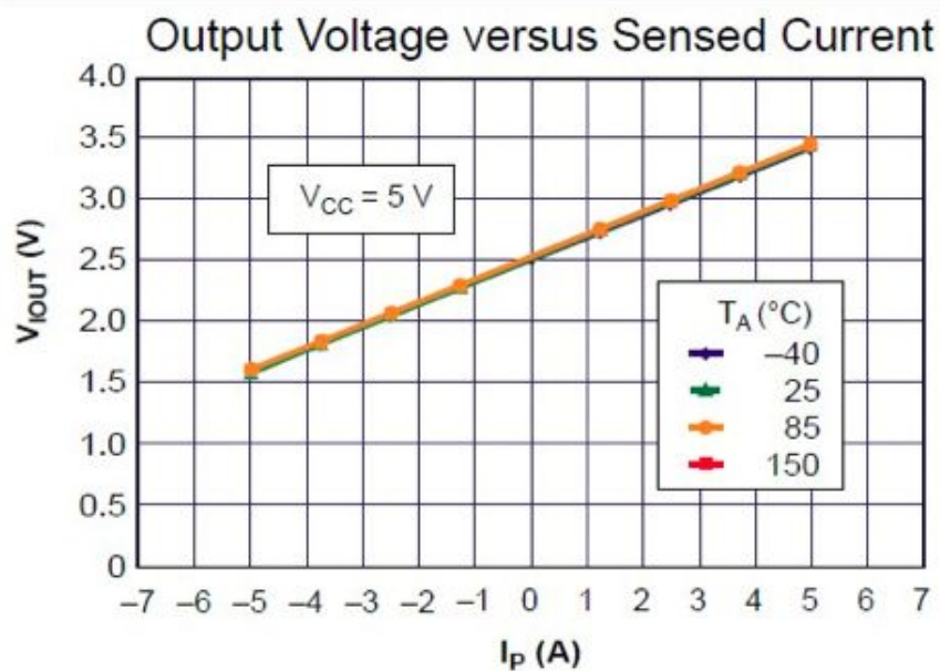
Figura 2.5: Relación lineal entre el Voltaje obtenido de salida del sensor y la Corriente sensada por el mismo. Fuente: Allegro Microsystems ACS712.
