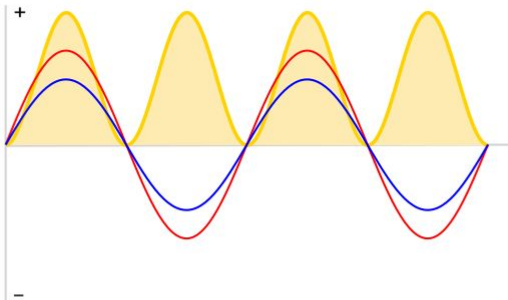
Figura 2.1: Relaciones de tensión y corriente en una carga puramente resistiva. En amarillo la potencia p(t) , en rojo el voltaje v(t) y en azul la corriente i(t) . Fuente: https://learn.openenergymonitor.org/electricity-monitoring/ac-power-theory/introduction .
