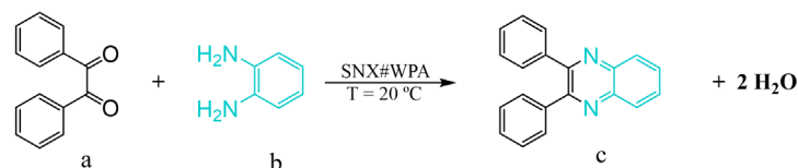
Figura 1. Síntesis de 2,3-difenilquinoxalina, DFQ (c), a partir de bencilo (a) y 1,2-fenildiamida (b).
