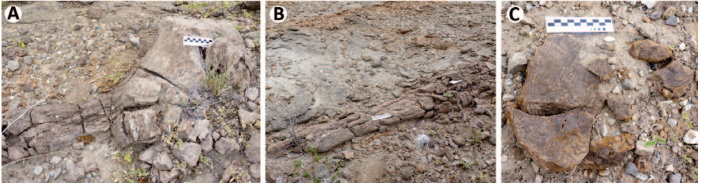
Figura 4: Troncos permineralizados preservados en la Formación Carrizal. a) Tocón de una gimnosperma en posición de vida, con parte de la raíz (NFII, Miembro Arroyo Seco); b) Resto de tronco de transportado que yace en sentido paralelo a la estratificación (NFIII, Miembro Rickard); c) Vista transversal de un tronco de Rhexoxylon cf. pianitzkyi (NFIV, Miembro Rickard).
