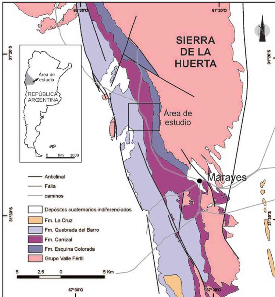
Figura 1: Mapa geológico (modificado de Bossi 1976) del área de estudio. En el recuadro se muestra la región donde se relevaron los perfiles sedimentológicos y los niveles fosilíferos de la Formación Carrizal.
