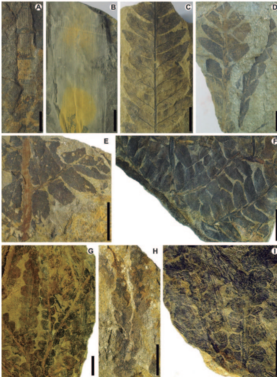
Figura 5: a) Equisetites fertilis (Frenguelli) Frenguelli 1944a, PBSJ 869; b) Neocalamites carrerei (Zeiller) Halle 1908, PBSJ 871; c) Cladophlebis mesozoica (Kurtz) Frenguelli 1947 PBSJ 888; d) Dicroidium odontopteroides (Morris) Gothan 1912, PBSJ 905; e) Cladophlebis kurtzi Frenguelli 1947, PBSJ 879; f) Cladophlebis mesozoica PBSJ 884; g-i) Dicroidium argenteum (Retallack) Gnaedinger y Herbst 2001; g) PBSJ 893, I, PBSJ 897; h) Johnstonia stelzneriana (Geinitz) Frenguelli 1943, PBSJ 908. Escala gráfica: 1 cm.
