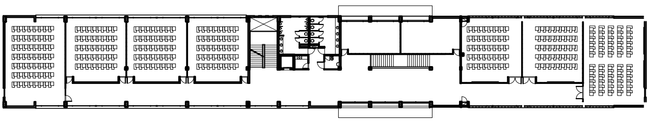
PLANTA 2º PISO
