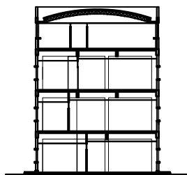
CORTE TRANSVERSAL
