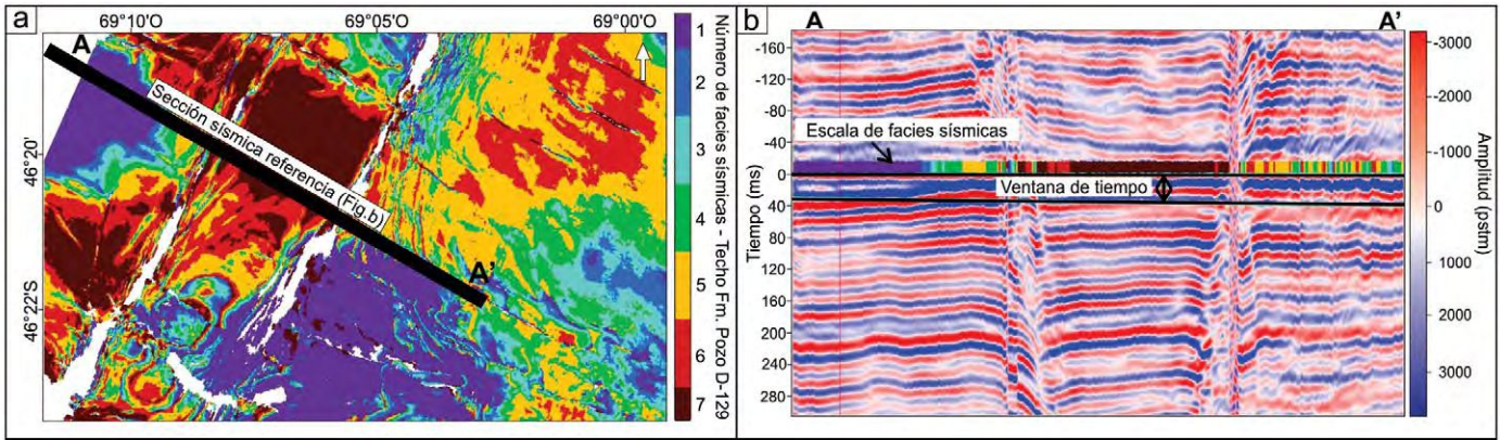
Figura 11: a) Mapa de facies sísmicas (1 a 7). b) Sección sísmica con ventana de trabajo y sobreimposición del mapa de facies sísmicas.
