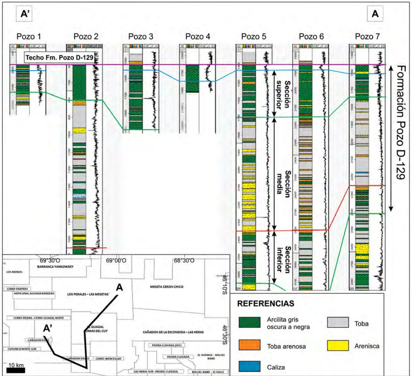
Figura 2: Corte estratigráfico de siete pozos exploratorios horizontalizados al techo de la Formación Pozo D-129. Se despliega el perfil sísmico (DT) y la columna litológica descrita por control geológico. Se discriminan las tres secciones de la unidad, descritas en el texto.
