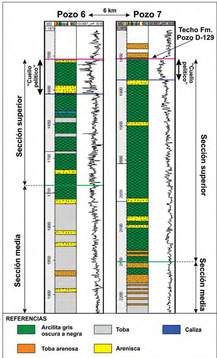
Figura 3: Litología y perfil sónico (DT) de los pozos en la zona de estudio en la que se focaliza la Sección Superior de la Formación Pozo D-129, el intervalo correspondiente al “cuello pelítico” y el techo de la sección media.
