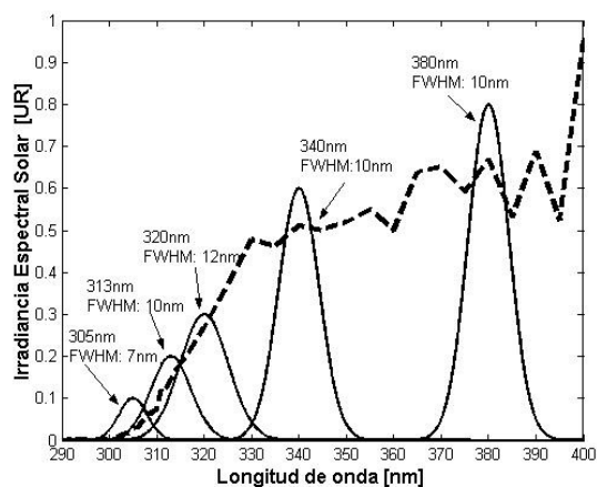
Figura 1: Representación esquemática de la ubicación y distribución espectral de los filtros de los 5 canales del Instrumento GUUV 541 de Biospherical Instrument.
