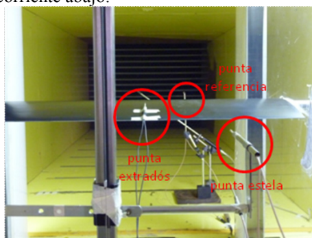
Figura 2. Disposición de los sensores de anemometría de hilo caliente.
