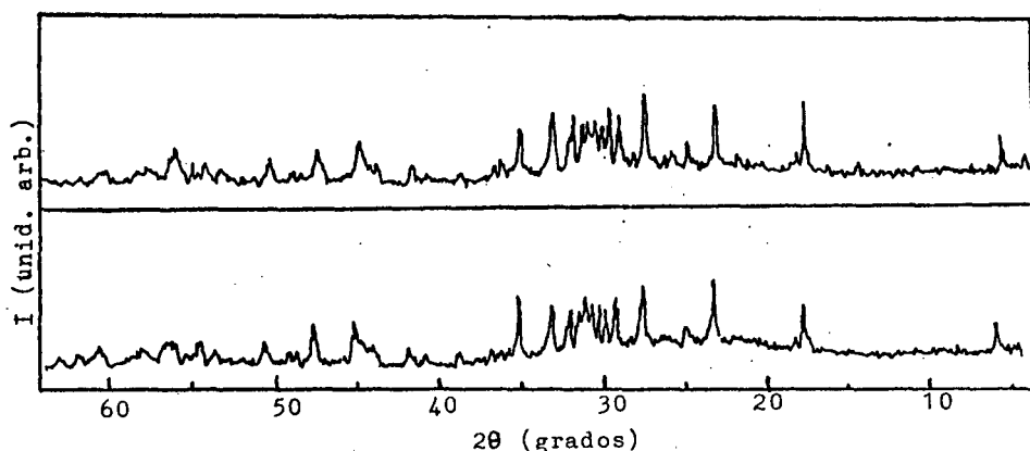
Figura 1: Difractograma de rayos X. Figura superior: muestra A. Figura inferior: muestra B
