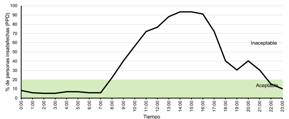
Figura 9. Gráfica de PPD (Porcentaje de personas insatisfechas) en el día típico. Fuente: elaboración propia (2019).
