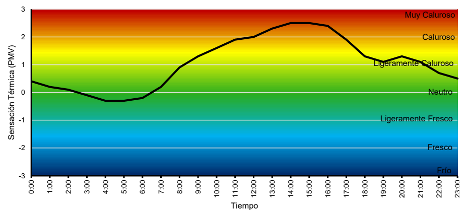
Figura 8. Gráfica de PMV (índice de sensación térmica) en el día típico. Fuente: elaboración propia.
