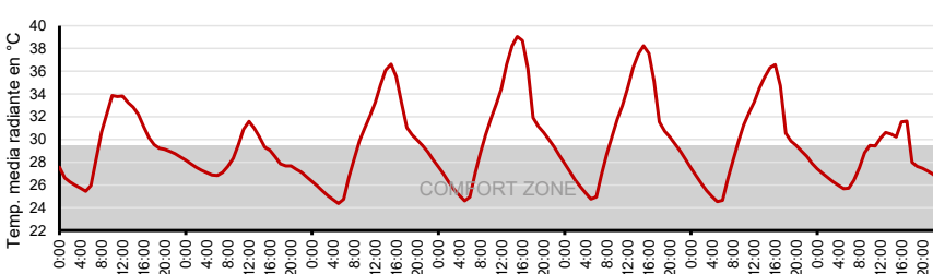
Figura 7. Temperatura media radiante durante los siete días de monitoreo.
