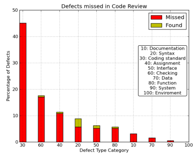
Figura 10: Distribución de Pareto de los defectos (fase compilación)
