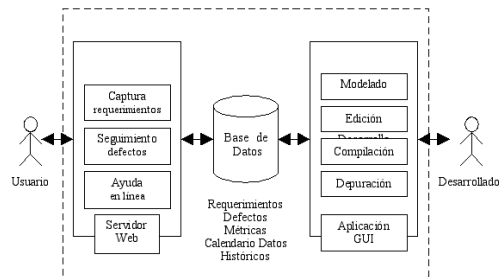
Figura 5: Esquema básico de la Herramienta I-CASE desarrollada
