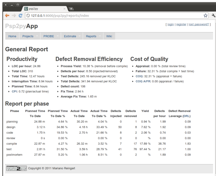
Figura 7: Captura de la página general de aplicación web (psp2py)
