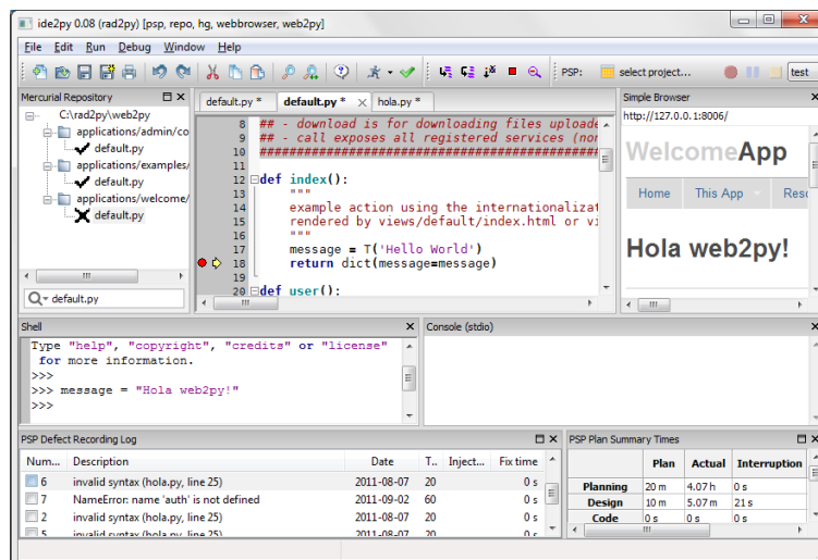
Figura 6: Captura de la pantalla principal de la IDE desarrollada (ide2py)
