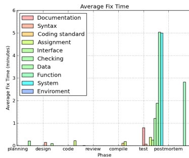
Figura 11: Tiempos promedio de corrección de errores
