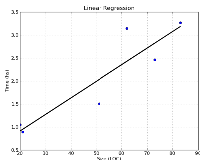
Figura 8: Regresión Lineal del tamaño (SLOC) y tiempos (en horas)
