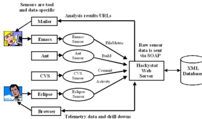
Figura 2: Esquema de Hackystat [9]
