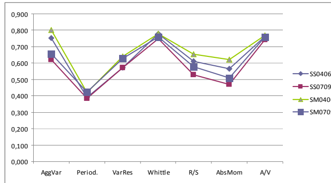
Figura 4: Comparación de las estimaciones del parámetro de HURST por SELFIS.
