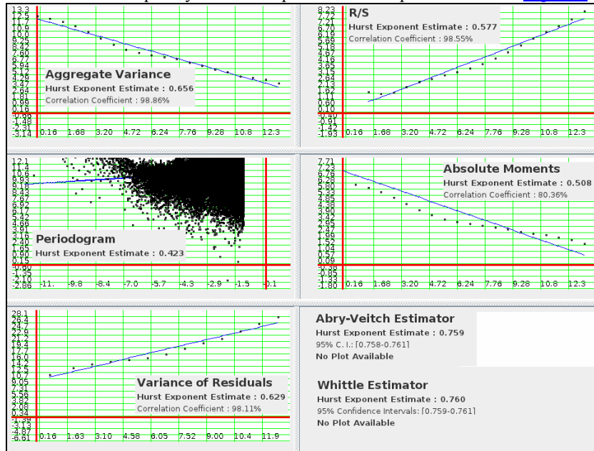
Figura 3: Estimación de Parámetro de HURST realizado con SELFIS
