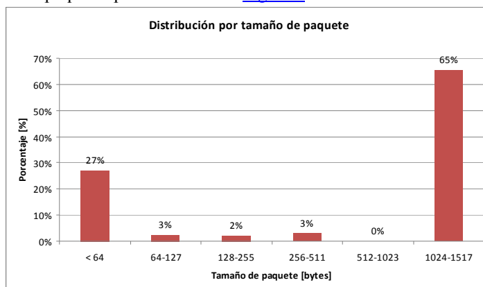
Figura 1: Distribución por Tamaño de Paquete.
