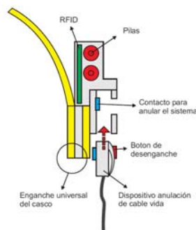
Figura 4 Dispositivo de seguro al cable vida
