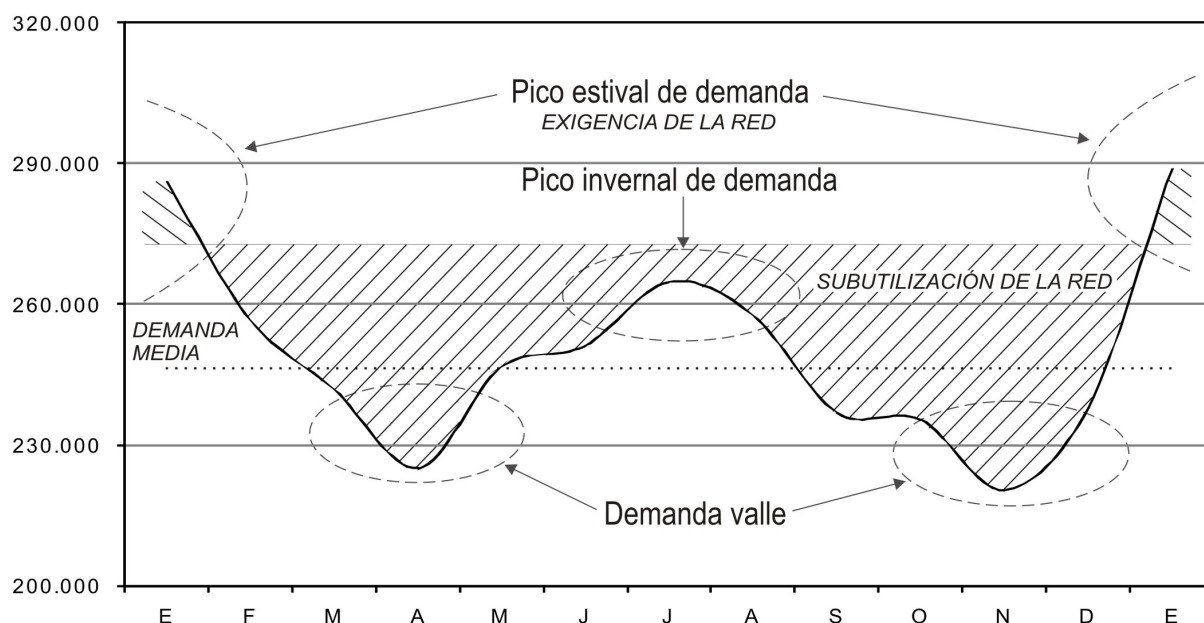
Figura 3. Demanda eléctrica media mensual de la región atlántica bonaerense (Mwh). El método de ajuste para la construcción de la serie se basa en el sencillo procedimiento de calcular cada una de las puntuaciones de la curva como la media aritmética de los valores mensuales de los respectivos años considerados. Por ejemplo: Demanda del mes de mayo = demanda de mayo 2007 + demanda de mayo 2008 + demanda de mayo 2009) / 3. Para calcular el valor del mes de enero que cierra el ciclo, respetando la progresión histórica, se incorporó excepcionalmente el dato de 2010. Fuente: elaboración personal con datos de CCA (2007-2010).
