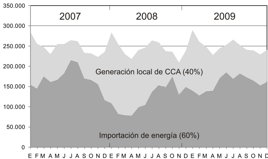
Figura 5. Cobertura de la demanda eléctrica de la región atlántica. 2007-2009. Fuente: elaboración personal con datos de CCA (2007-2010)
