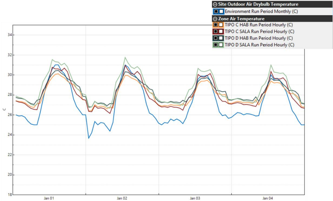
Gráfica 27. Comportamiento térmico espacios Apartamento Tipo C y Tipo D. Propuesta
