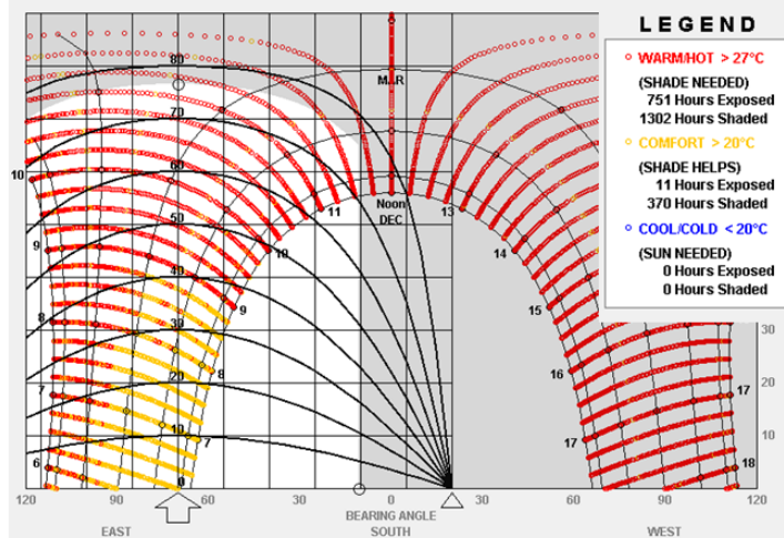
Figura 22. Diagnóstico de sombra en ventana pequeña retrocedida fachada sureste
