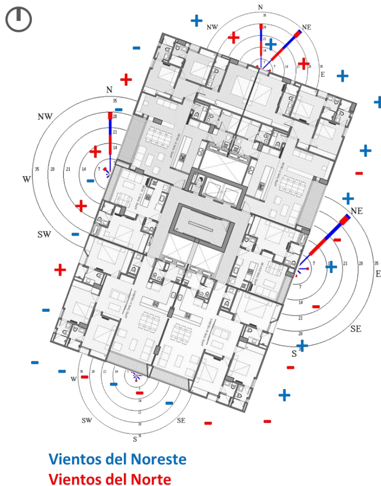
Figura 50. Esquema de presiones de viento en el proyecto
