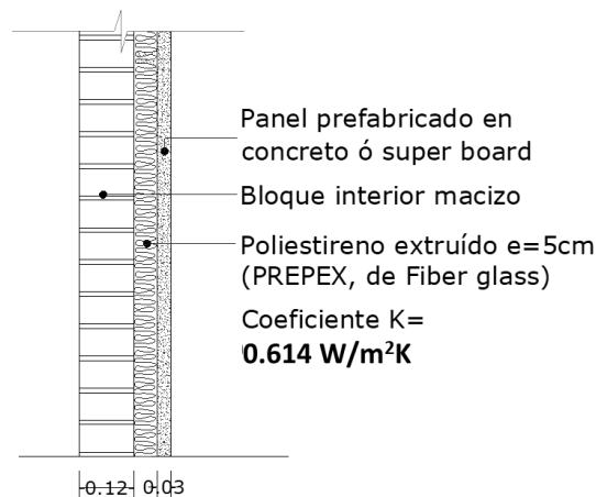
Figura 48. Detalle muro propuesto. Elaboración propia
