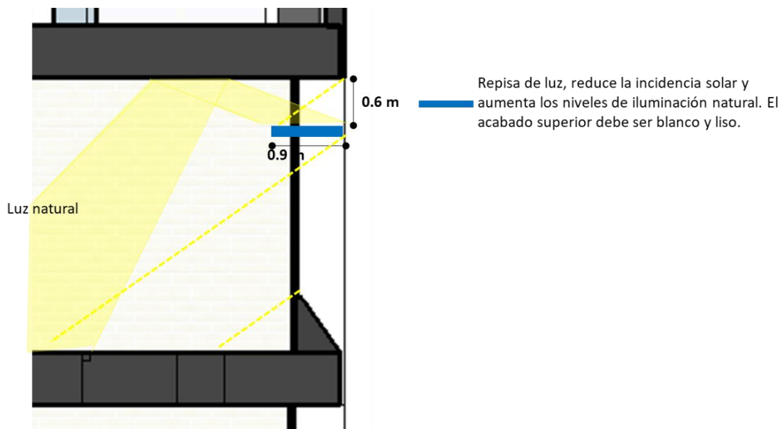
Figura 45. Propuesta de protección solar fachada noroeste - ventana pequeña
