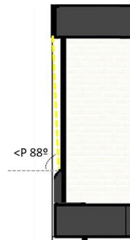
Figura 23. Diagnóstico de sombra en ventana pequeña con poco retroceso fachada sureste
