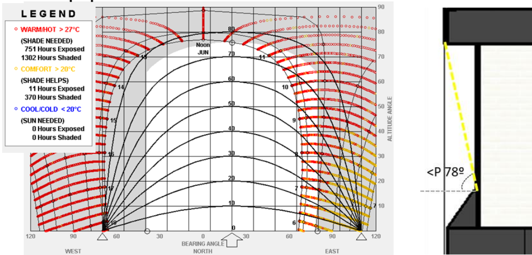
Figura 30. Diagnóstico de sombra en ventana pequeña retrocedida fachada noreste
