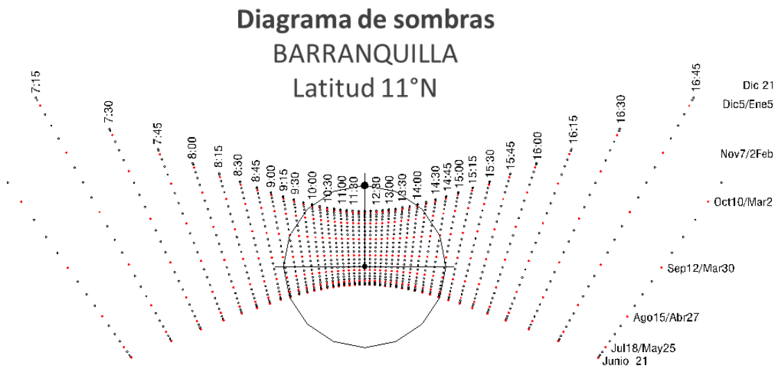
Figura 14. Diagrama de sombra Barranquilla. Fuente: PVG Arquitectos.
