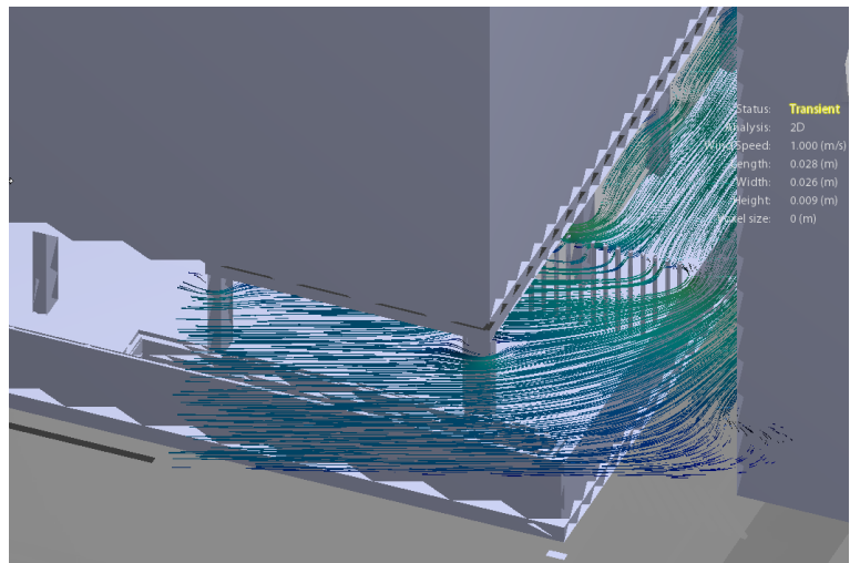
Figura 62. Simulación aerodinámica espacio de piscina. Zoom barrera permeable
