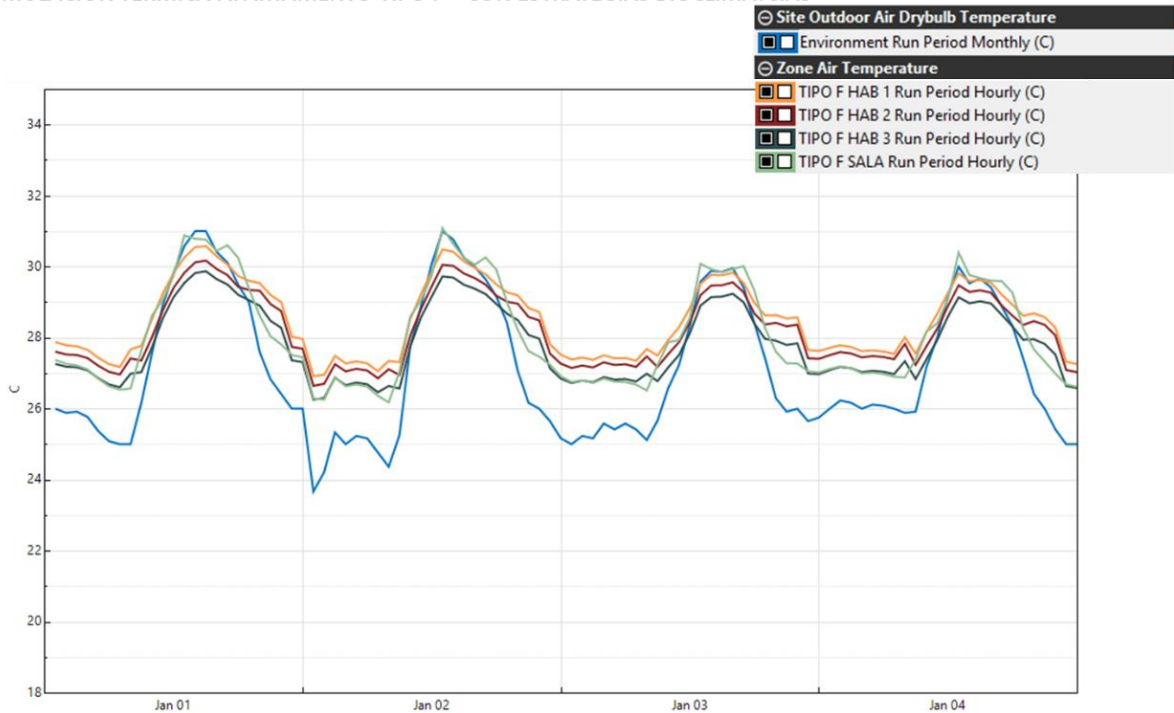
Gráfica 29. Comportamiento térmico espacios Apartamento Tipo F. Propuesta
