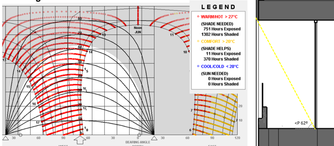
Figura 29. Diagnóstico de sombra en balcón grande fachada noroeste
