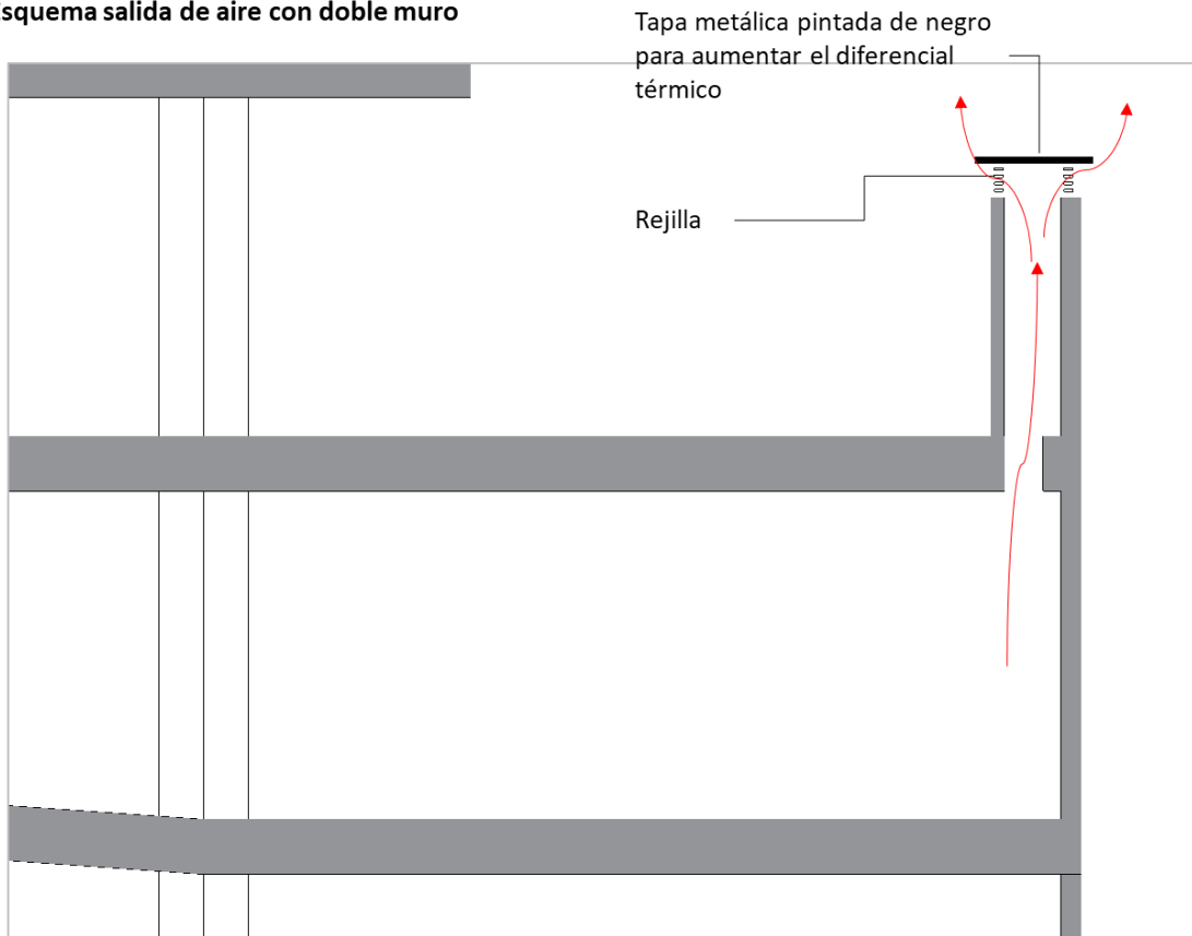
Figura 58. Esquema de salida de aire por efecto stack
