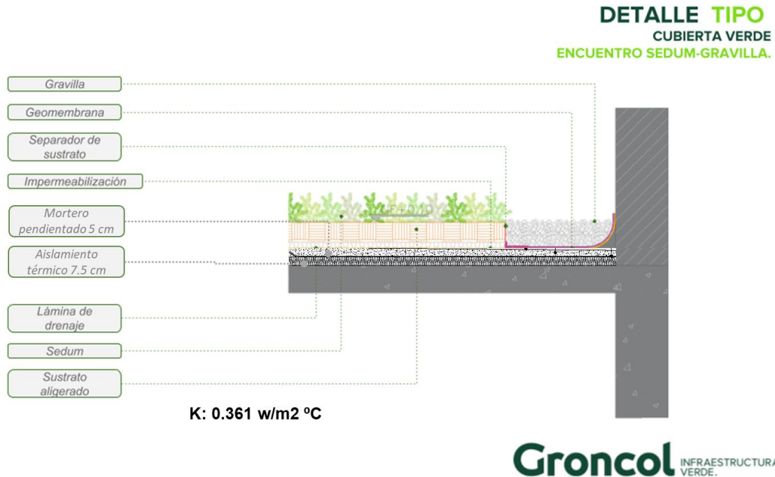
Figura 47. Detalle cubierta . Elaboración propia a partir de detalle enviado por empresa Groncol
