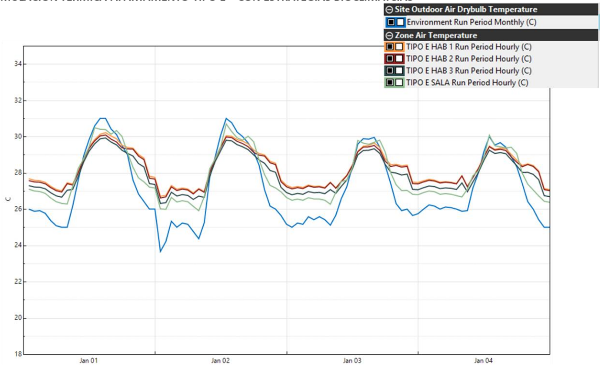
Gráfica 28. Comportamiento térmico espacios Apartamento Tipo E. Propuesta
