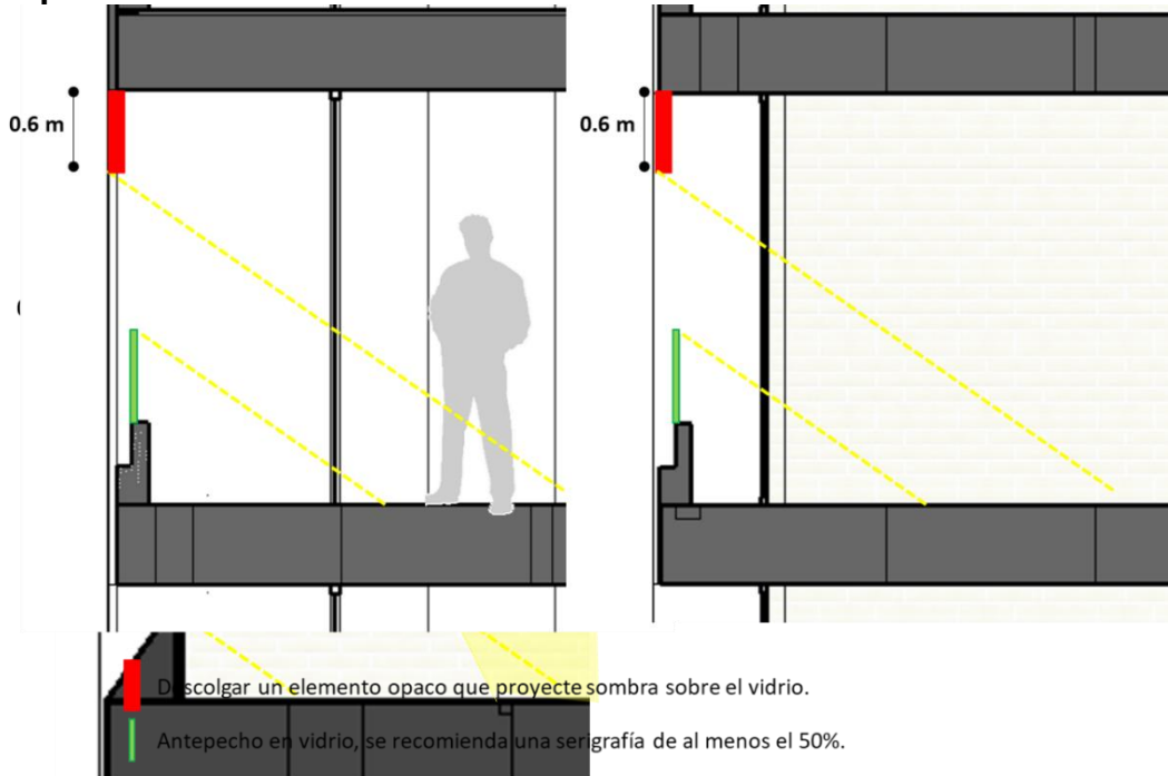
Figura 42. Propuesta de protección solar fachada sureste
