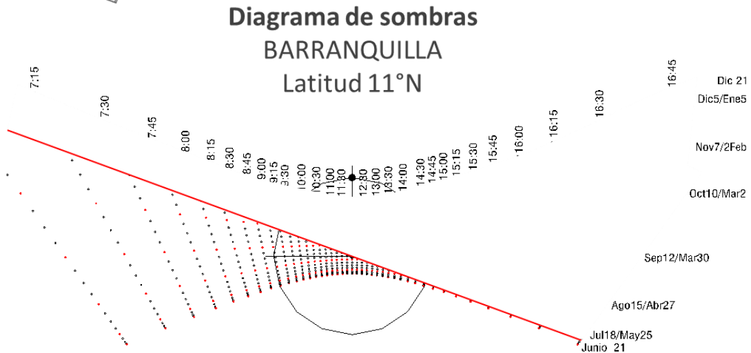
Figura 15. Análisis fachada noreste mediante diagrama de sombras. Elaboración propia
