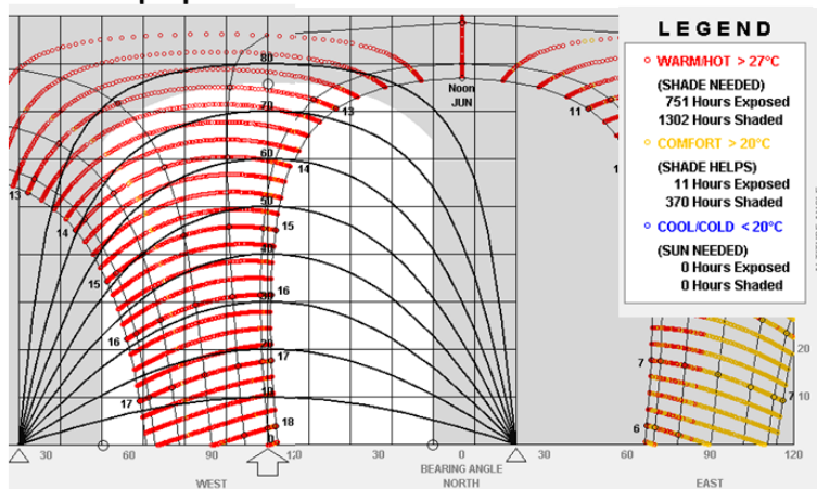
Figura 26. Diagnóstico de sombra en ventana pequeña retrocedida fachada noroeste
