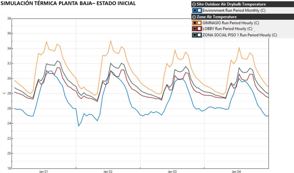
Gráfica 13. Comportamiento térmico espacios Planta Baja. Estado Inicial
