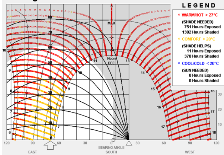
Figura 25. Diagnóstico de sombra en balcón grande fachada sureste
