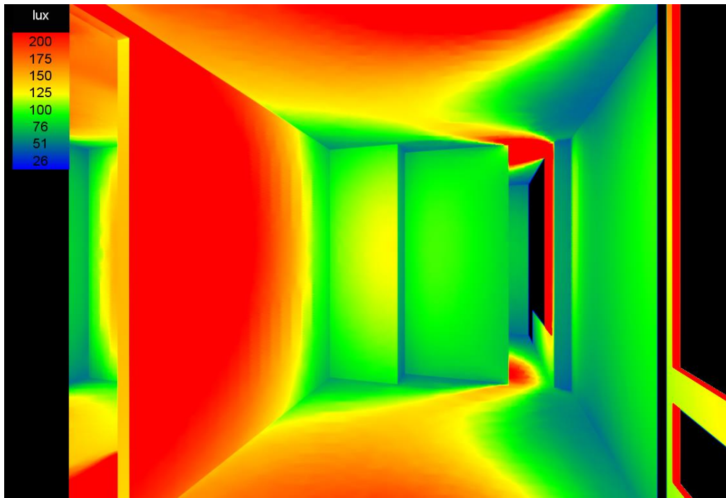
Figura 65. Simulación lumínica en perspectiva de un espacio de habitación
