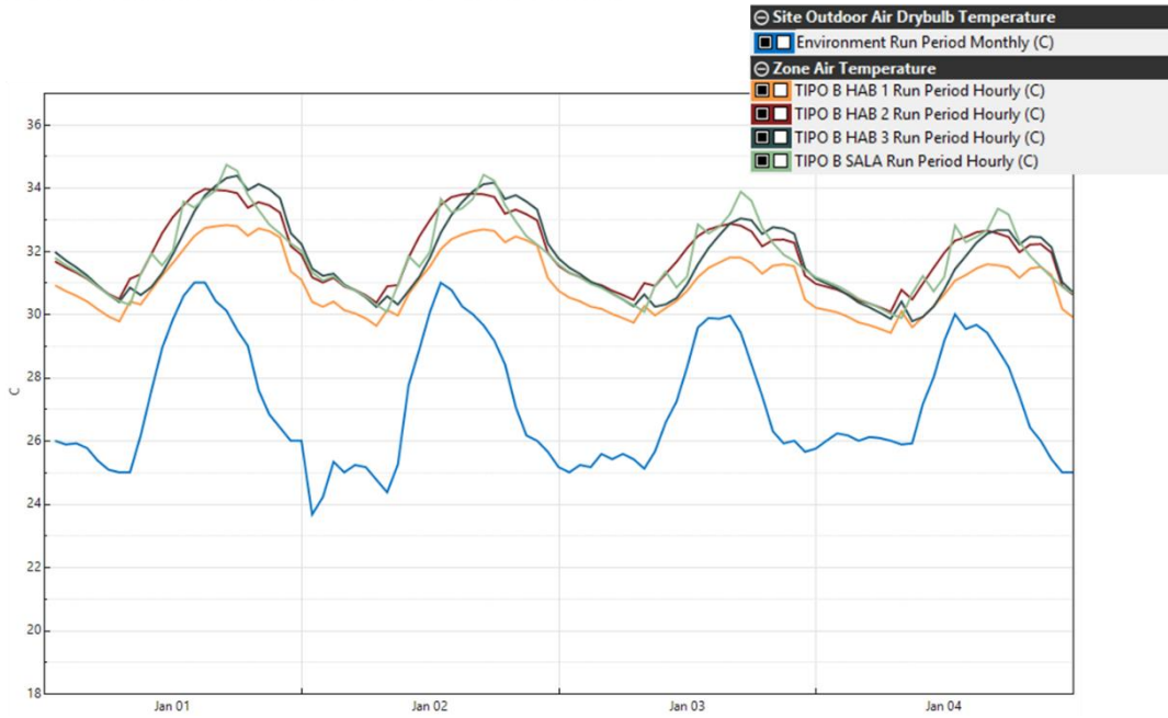
Gráfica 17. Comportamiento térmico espacios Apartamento Tipo B. Estado Inicial
