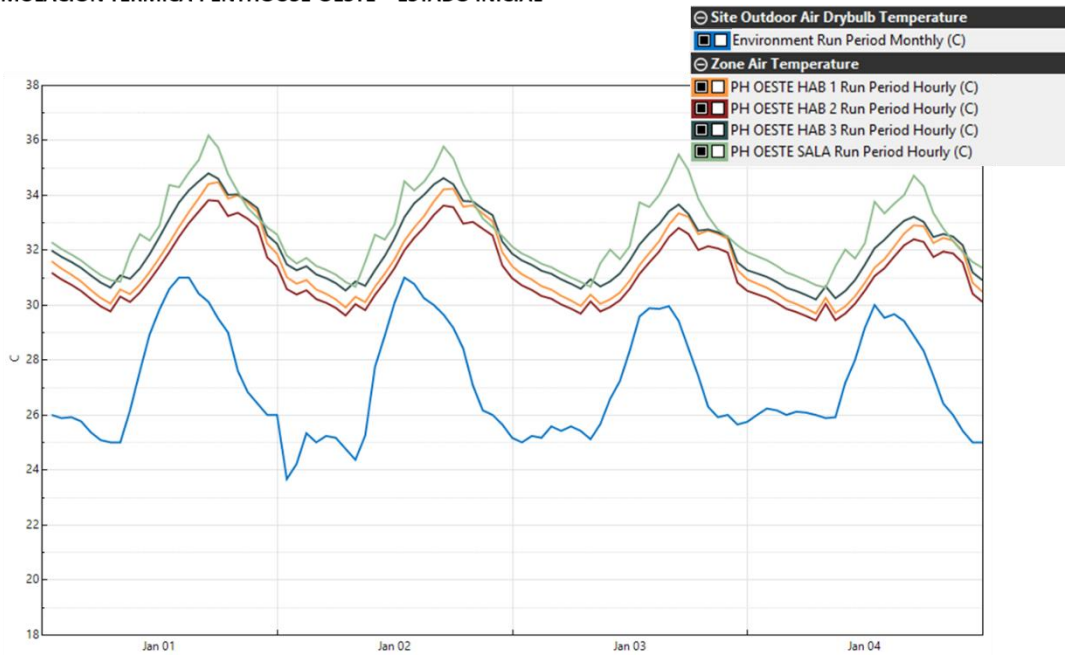
Gráfica 15. Comportamiento térmico espacios del Penthouse Oeste. Estado Inicial
