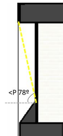
Figura 26. Diagnóstico de sombra en ventana pequeña retrocedida fachada noroeste
