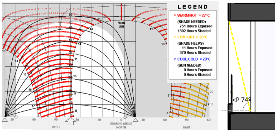
Figura 28. Diagnóstico de sombra en balcón pequeño fachada noroeste
