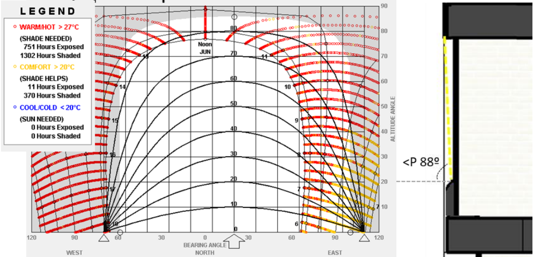
Figura 31. Diagnóstico de sombra en ventana pequeña con poco retroceso fachada noreste
