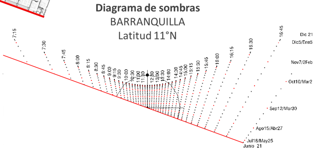
Figura 16. Análisis fachada suroeste mediante diagrama de sombras. Elaboración propia
