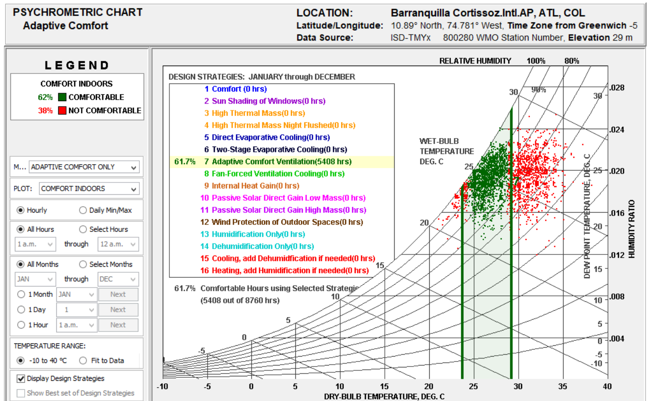
Gráfica 11. Cuadro Psicrométrico clima Barranquilla - Confort adaptativo. Fuente: Climate Consultant. 2016
