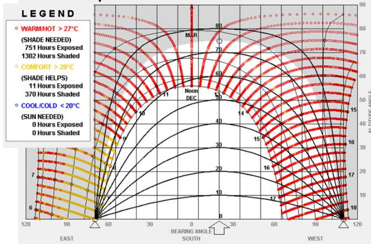
Figura 21. Diagnóstico de sombra en balcón último piso fachada suroeste
