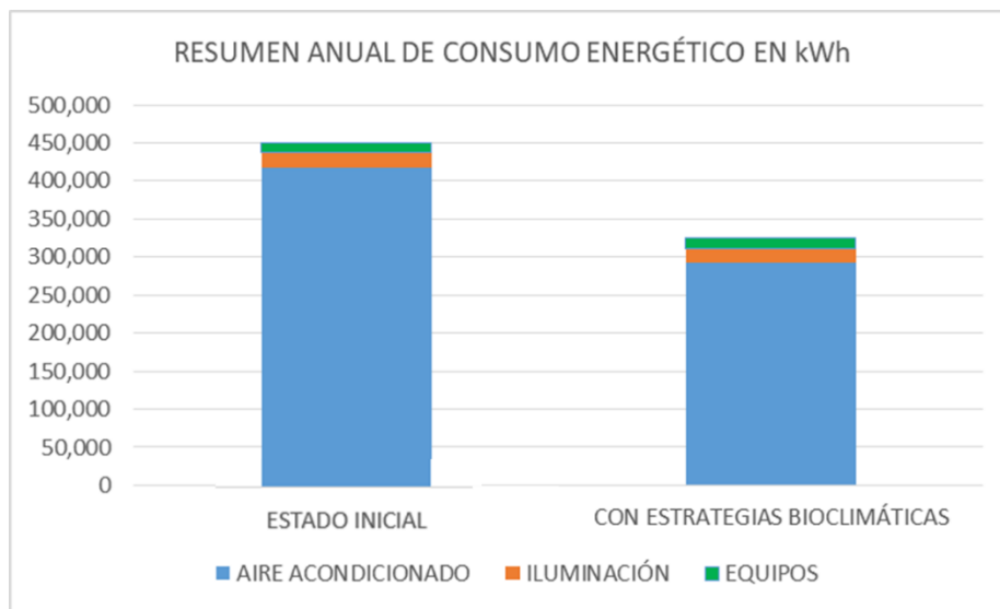
Gráfica 31. Comparativo resumen anual de consumo energético. Propuesta inicial y modelo mejorado
