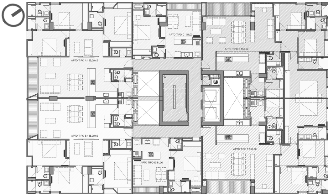
Figura 10. Piso tipo - Planta apartamentos del piso 1 al 7
