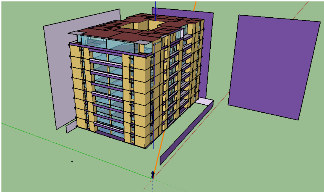
Figura 63. Modelo geométrico con propuestas en OpenStudio
