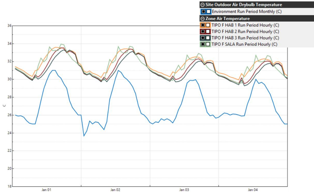
Gráfica 20. Comportamiento térmico espacios Apartamento Tipo F. Estado Inicial
