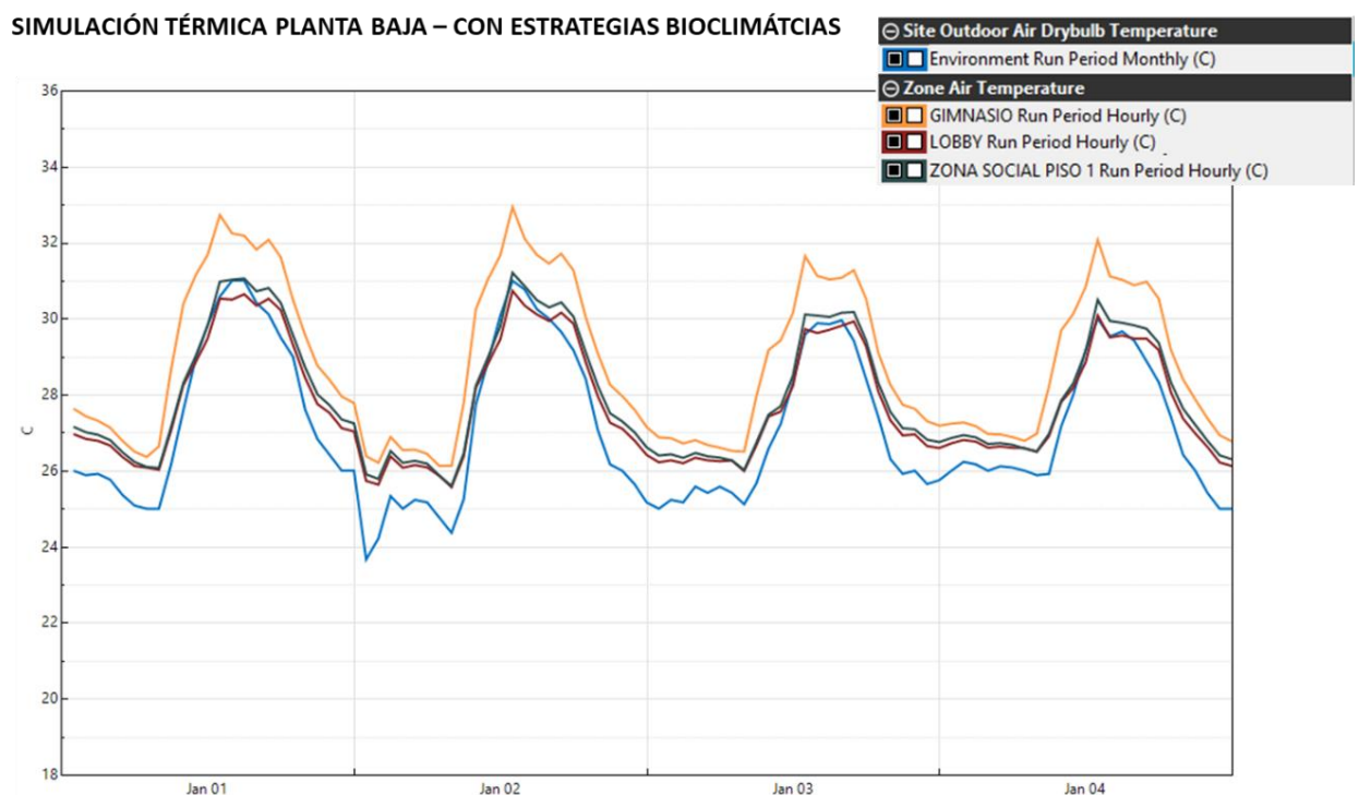
Gráfica 22. Comportamiento térmico espacios Planta Baja. Propuesta
