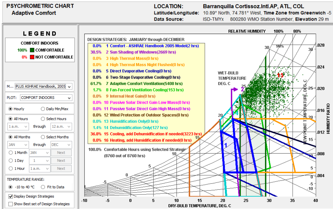
Gráfica 12. Cuadro Psicométrico clima de Barranquilla - Estrategias a aplicar. Fuente: Climate Consultant. 2016
