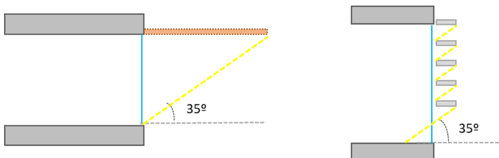
Figura 40. Ejemplo de aplicación de los ángulos de protección solar
