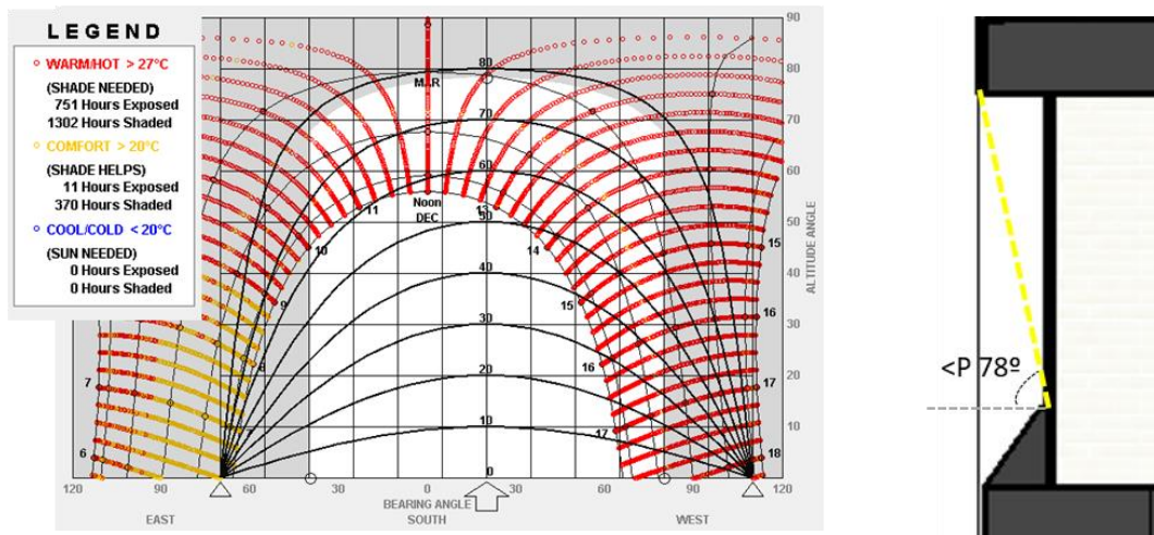
Figura 19. Diagnóstico de sombra en ventana pequeña retrocedida fachada suroeste
