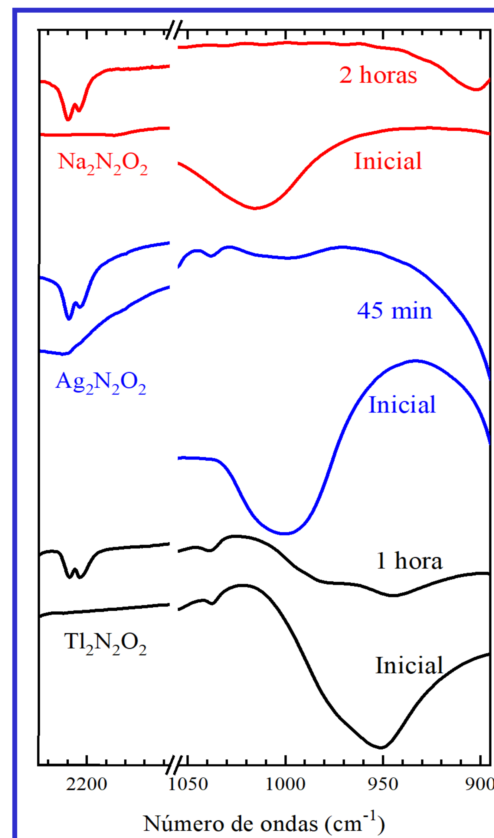
Figura 2. Espectros de infrarrojo de los hiponitrito de sodio, plata y talio antes y después de la irradiación con luz de \lambda = 253,7 nm, (a) Na_2N_2O_2 , (b) Ag_2N_2O_2 , (c) Tl_2N_2O_2
