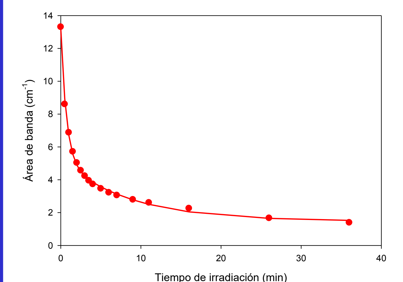
FIGURA 4. Cinética de descomposición del Tl_2N_2O_2 en función del tiempo de irradiación con luz proveniente de una lámpara de mercurio de baja presión (principalmente \lambda = 253,7 nm).
