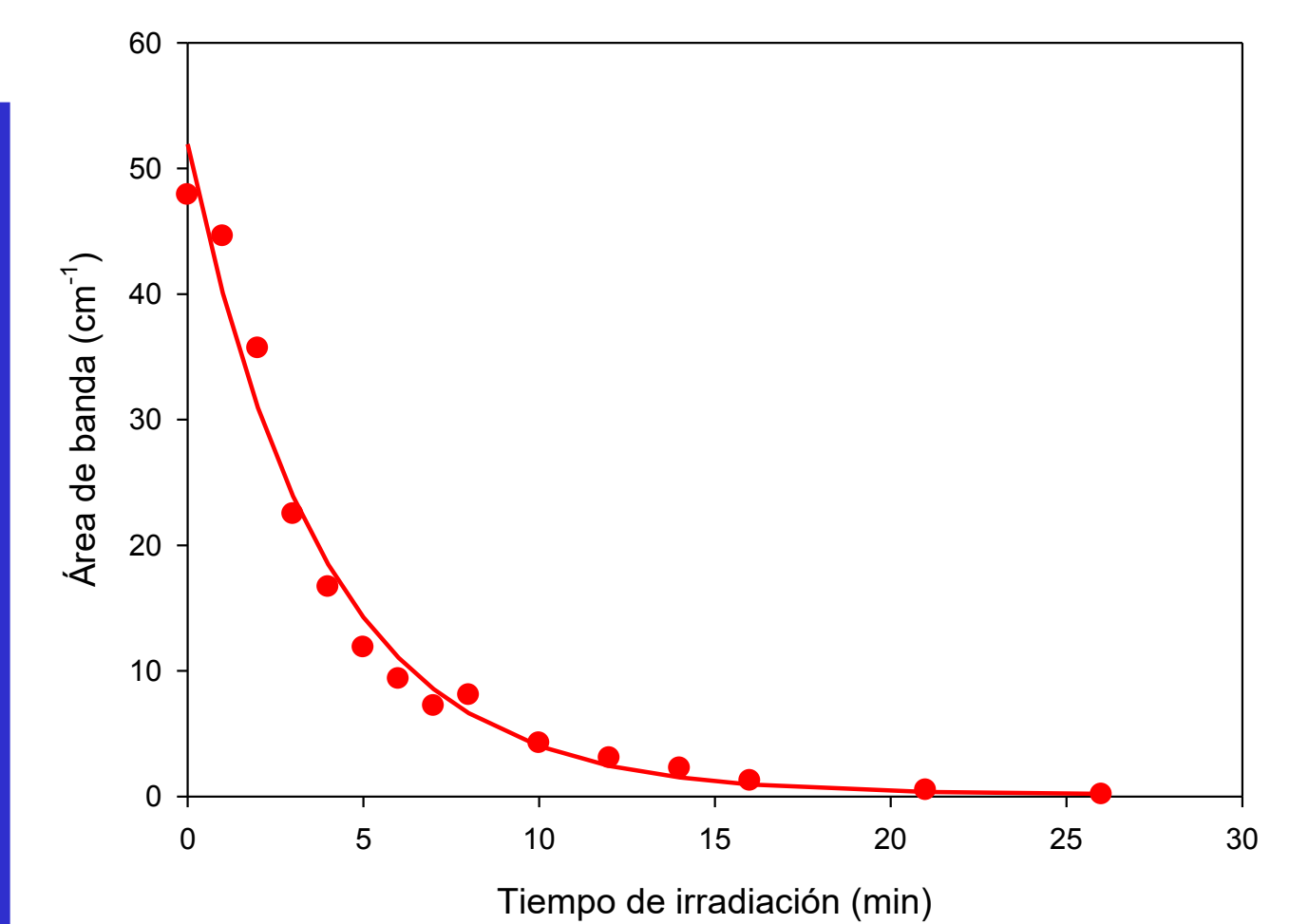
FIGURA 3. Cinética de descomposición del Na_2N_2O_2 en función del tiempo de irradiación con luz proveniente de una lámpara de mercurio de baja presión (principalmente \lambda = 253,7 nm)
