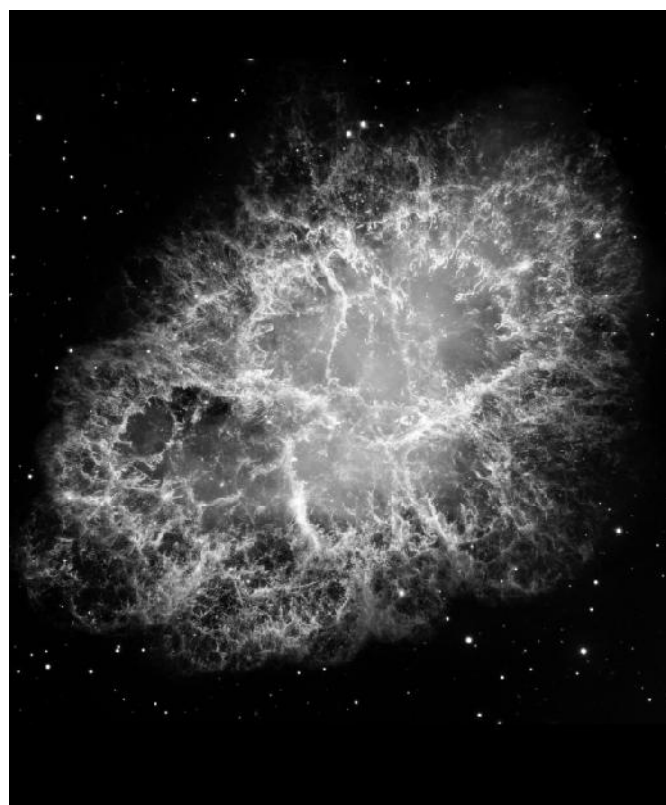
Figura 6: Nebulosa del Cangrejo, los restos de la SN1054, en nuestra galaxia. Crédito: NASA y ESA.
