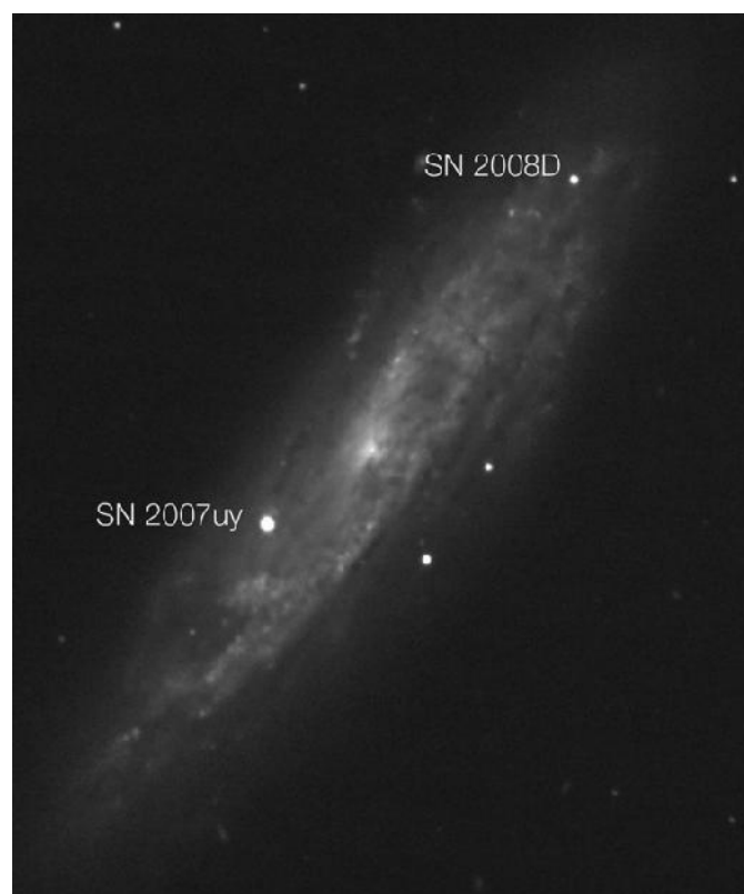
Figura 4: Supernovas en la galaxia NGC 2770. La sigla NGC se debe al Nuevo Catálogo General, una compilación enorme de objetos celestes difusos. Imagen: European Southern Observatory
