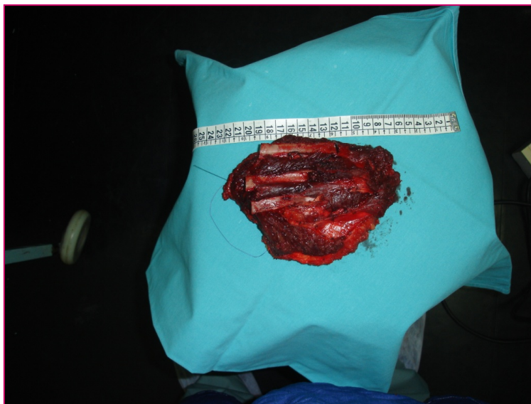
PIEZA OPERATORIA
