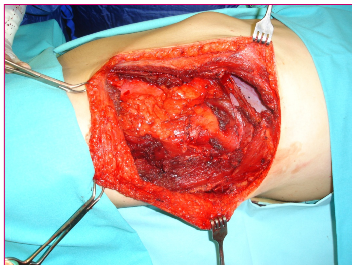
LECHO QUIRÚRGICO
