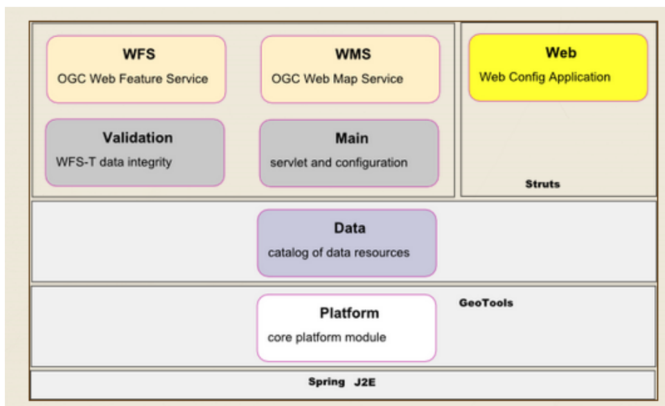
Figura 8: Arquitectura modular de GeoServer
