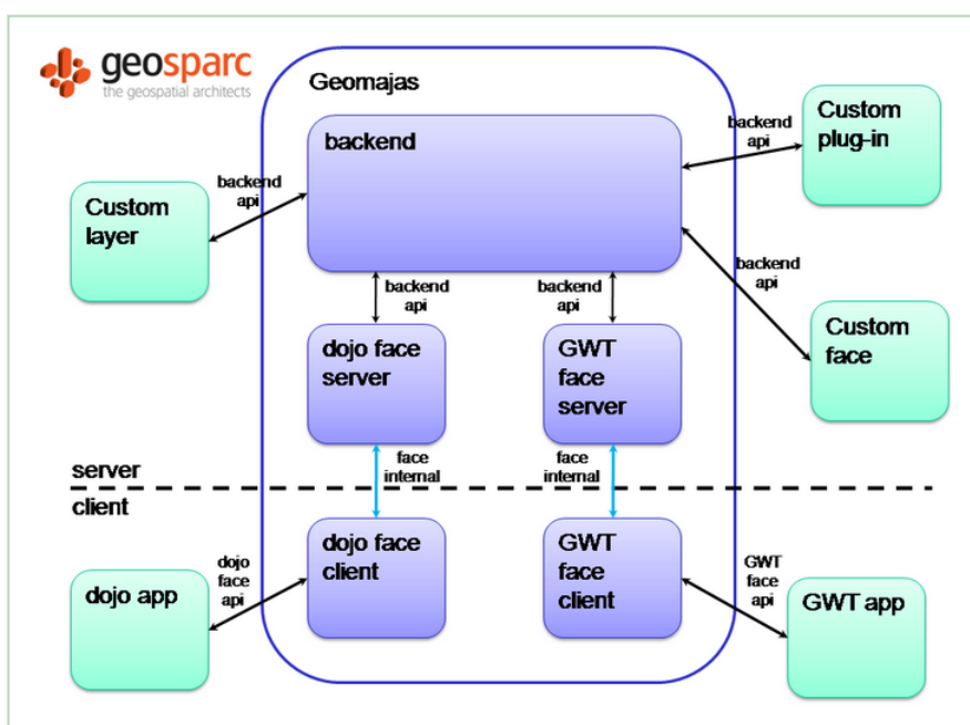
Figura 9: Arquitectura de Geomajas, extraído de "Geomajas user guide for developers" capítulo Architecture
