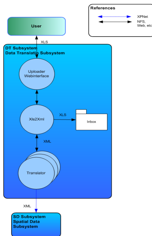
Figura 3: El subsistema DT
