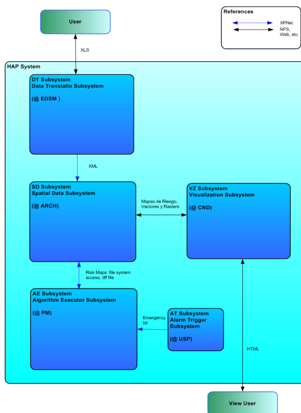
Figura 2: Representación arquitectural del sistema SAT/ERDNU.
