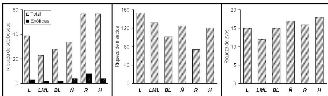
Gráfico 2. Riqueza del sotobosque, insectos y aves en ambientes asociados.
