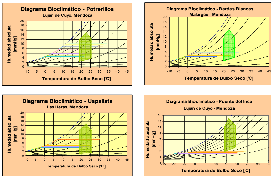
Figura 1: diagramas bioclimáticos correspondientes a las localidades en estudio.
