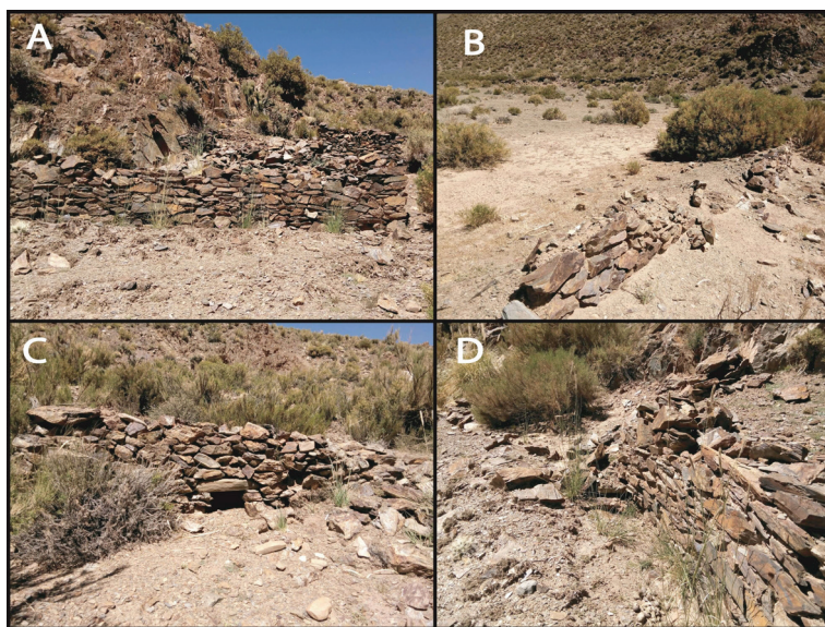
Figura 5. Vistas de la andenería del sector superior de Matancillas; (a) muro canteado; (b) pared; (c) boca de canal de riego; (d) muro de contención de andenería
